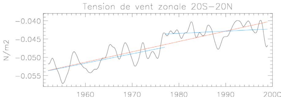
Figure 4.5.b : Variations interannuelles (en \text{N.m}^{-2} ) de la tension de vent zonale NCEP moyenne du Pacifique tropical (en noir), tendances linéaires sur la période 1951-99 (en rouge) et sur les périodes 1951-76 et 1977-99 (en bleu).
