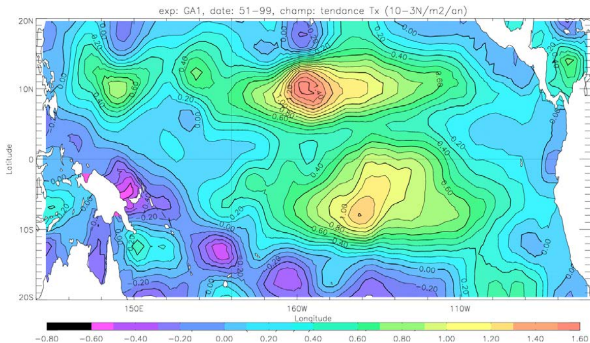
Figure 4.5.c : Tendence linéaire (en 10^{-3} \cdot \text{N.m}^{-2} \cdot \text{an}^{-1} ) de la tension de vent zonale NCEP sur la période 1951-99.
