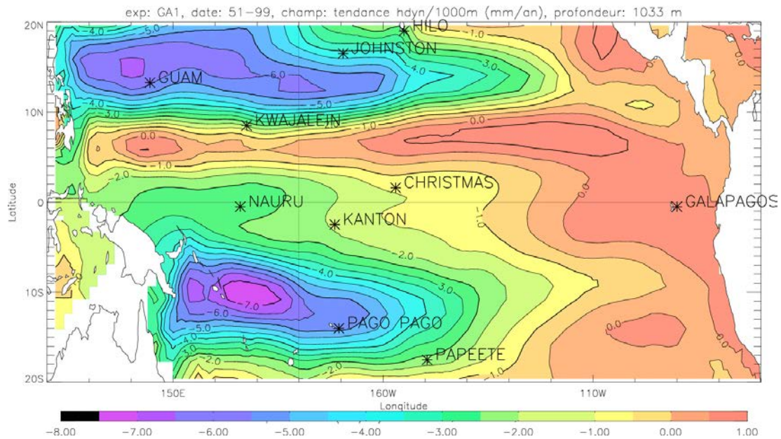
Figure 4.2.b : Tendance linéaire ( \text{mm.an}^{-1} ) en hauteur dynamique (référéncée à 1000 m) dans le modèle. Les marégraphes utilisés précédemment pour la validation sont indiqués (*).
