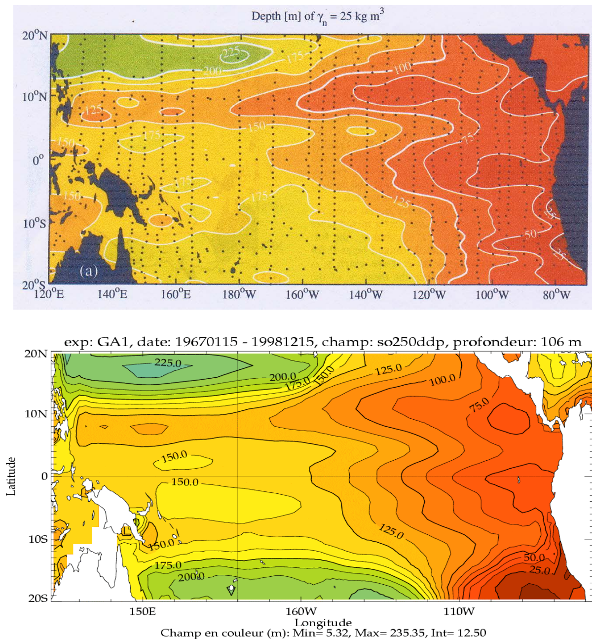
Figure 5.1.a : Profondeur moyenne (m) sur la période 1967-98 de l'isopycne \sigma_\theta = 25 \text{ kg.m}^{-3} caractéristique de la pycnocline, calculée par Johnson et McPhaden [1999] à partir des données CTD (en haut) et simulée par le modèle OPA (en bas). Les points noirs sur la figure du haut indiquent la position des profils hydrographiques utilisés. Noter que les palettes de couleurs diffèrent légèrement entre les deux cartes. Les isolignes sont espacées de 25 m sur la carte du haut et de 12.5 m sur la carte du bas pour mieux discerner les structures simulées.
