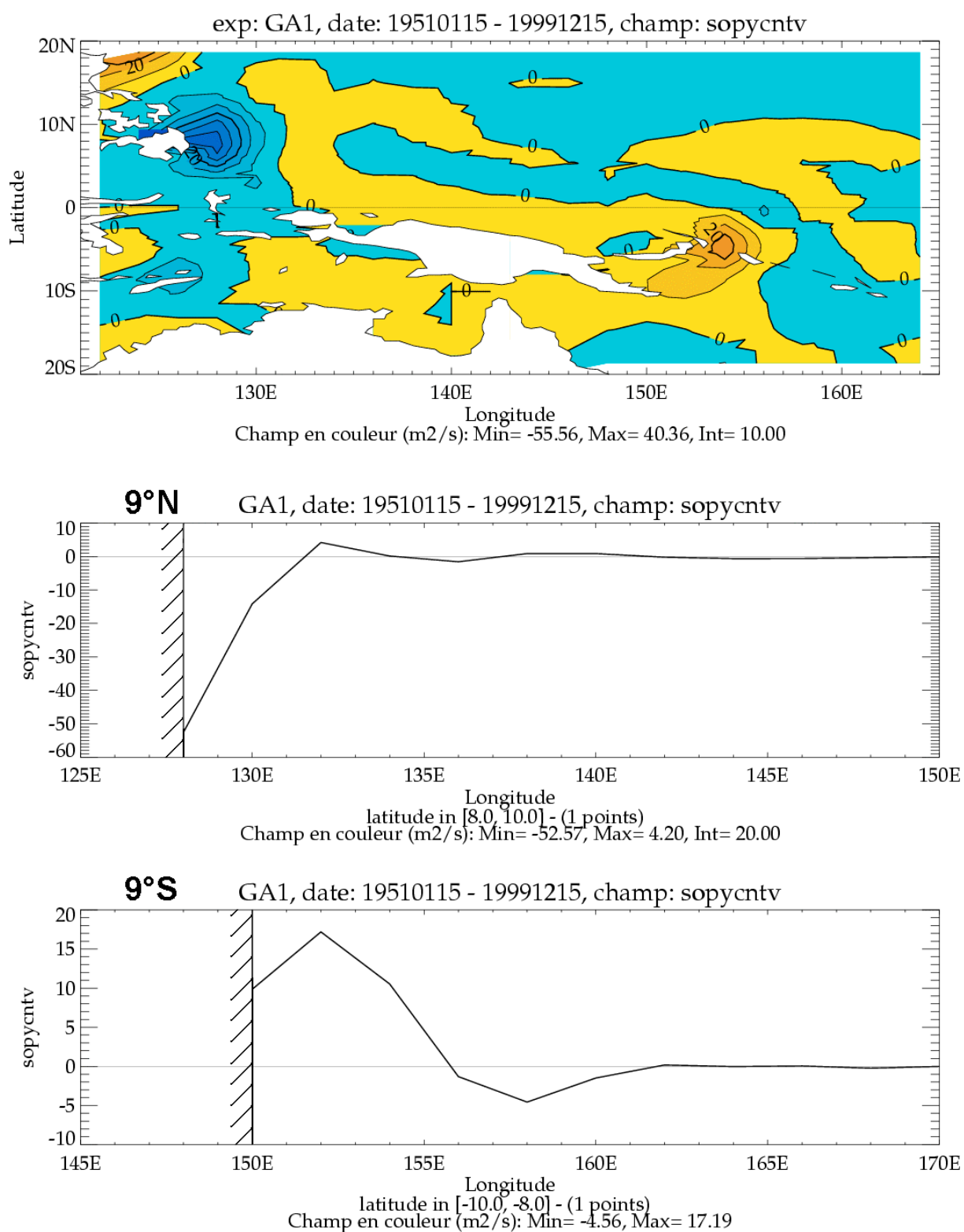
Figure 5.2.c : Transports moyens ( \text{m}^2 \cdot \text{s}^{-1} ) sur la période 1951-99 associés à la branche inférieure des STCs dans le Pacifique tropical ouest (en haut), et le long de 9°N (au milieu) et 9°S (en bas). Les valeurs positives indiquent les transports orientés vers le sud, les valeurs négatives les transports orientés vers le nord.
