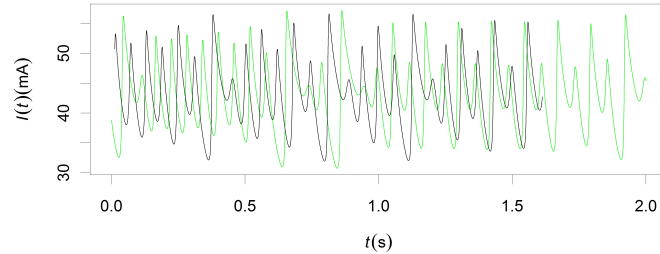
FIGURE 3.5 – Fenêtre sélectionnée d'un enregistrement d'intensité de courant I(t) mesuré lors d'une expérimentation d'électrolyse du cuivre dans de l'acide phosphorique obtenu par le groupe de John Hudson [71]. Ces données sont mises à disposition sur le site Web d' atomosyd ( http://www.atomosyd.net/ ).
