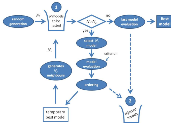
FIGURE 2.1 – Schéma de fonctionnement de l’algorithme PoMoS : (1) un ensemble de N_0 modèles initiaux est généré aléatoirement et mis dans le panier 1, (2) si le nombre de modèle est assez grand ( N > N_1 ), N_1 modèles sont testés sur la base d’un critère choisi de type Akaike C^{AIC} [62], (3) les meilleurs modèles sont sélectionnés, tandis que les mauvais sont rejetés dans le panier 2; (4) le meilleur modèle est utilisé pour générer N_2 modèles voisins qui sont ajoutés dans le panier 1 (une distance intermodèle est définie à cet effet). (5) Les étapes (2) à (4) sont répétées jusqu’à ce que le nombre de modèles dans le panier 1 devienne trop faible ( N \leq N_1 ); (6) la recherche de modèles est alors stoppée.
