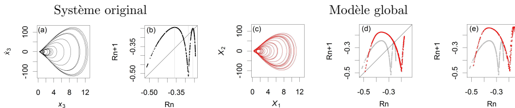
FIGURE 3.4 – Portraits de phase et applications de premier retour issus de la variable z du système Rössler (1 re et 2 e colonnes) puis issus du modèle global 30-termes (colonnes 3 à 5), la dernière applications de premier retour étant obtenue après l’ajustement manuel d’un paramètre.
