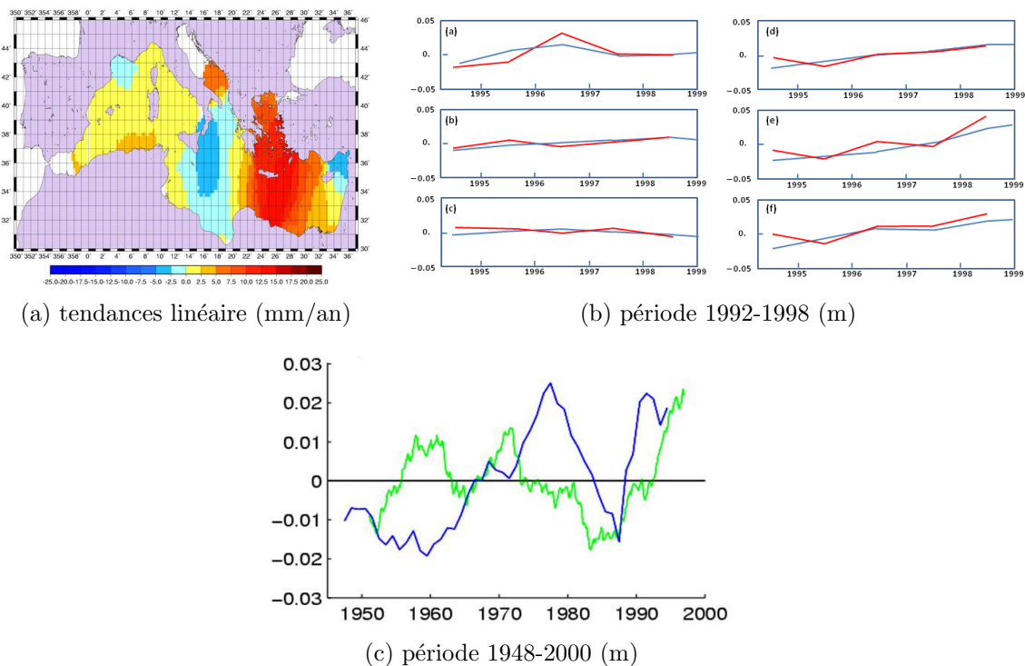
FIGURE 1.3 – Contribution thermostérique aux variations du niveau de la mer sur la période 1992-1998 en mer Méditerranée. Tendances linéaires en mm/an (a) ; séries temporelles de la contribution thermostérique et des variations observées dans six sous-régions (b) et dans le bassin occidental (c) méditerranéen.
