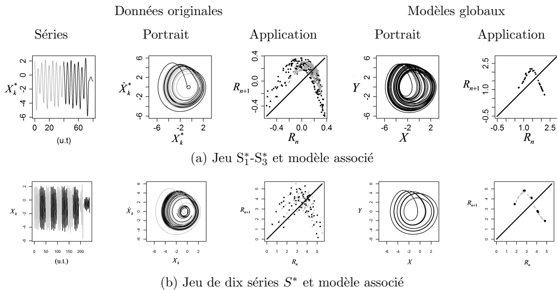
FIGURE 3.12 – Modèles globaux obtenus à partir de séries temporelles analysées en association et produites par des ensembles de systèmes de Rössler en synchronisation de phase avec un système de référence. Les colonnes sont structurées comme pour la Fig. 3.11.
