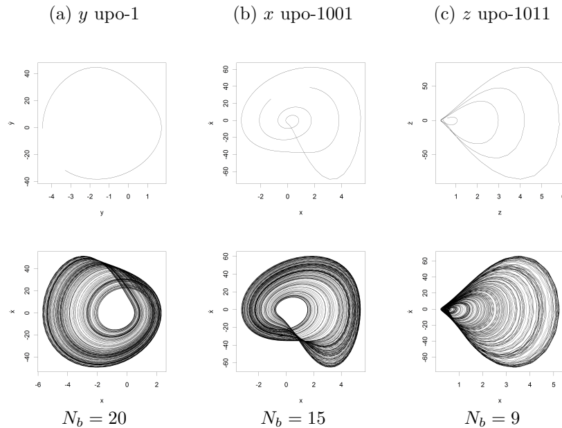
FIGURE 3.16 – Portraits de phase d'orbites périodiques instables utilisées comme série d'entrée (ligne du haut) et des modèles globaux correspondants obtenus pour chacune de ces séries (ligne du bas) issues de y , x et z . Les résultats sont présentés par degré décroissant d'observabilité (de gauche à droite) : (a) à partir de la variable y orbite (1); (b) à partir de la variable x orbite (1001); et (c) à partir de la variable z orbite (1011). N_b correspond à la taille des modèles globaux obtenus (nombre de termes).
