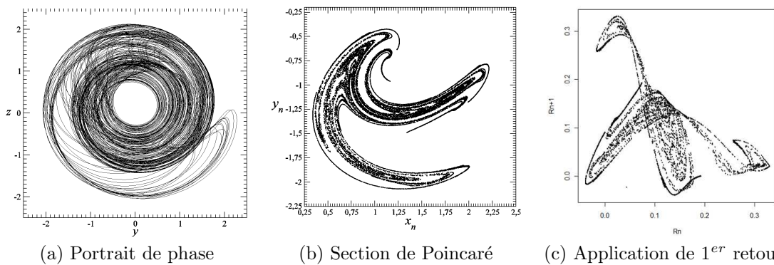
FIGURE 5.4 – Attracteur chaotique de structure toroïdale obtenu par intégration numérique des équations du système de Lorenz-84 (5.9). D_{KY} = 2.39 .
