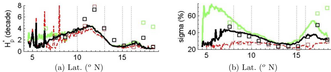
FIGURE 1.9 – Valeurs moyennes de l'horizon de prévisibilité H_P , et du pourcentage de bruit Gaussien \sigma en fonction de la latitude, pour une résolution de 8 \times 8 \text{ km}^2 (lignes pleines et pointillés) et pour une résolution de 128 \times 128 \text{ km}^2 (carrés). À noter que pour la résolution la plus basse de 1024 \times 1024 \text{ km}^2 , les valeurs H_P = 4.1 décades et \sigma = 24\% sont obtenues. Le lecteur est renvoyé à la publication originale pour une interprétation détaillée des courbes [7].
