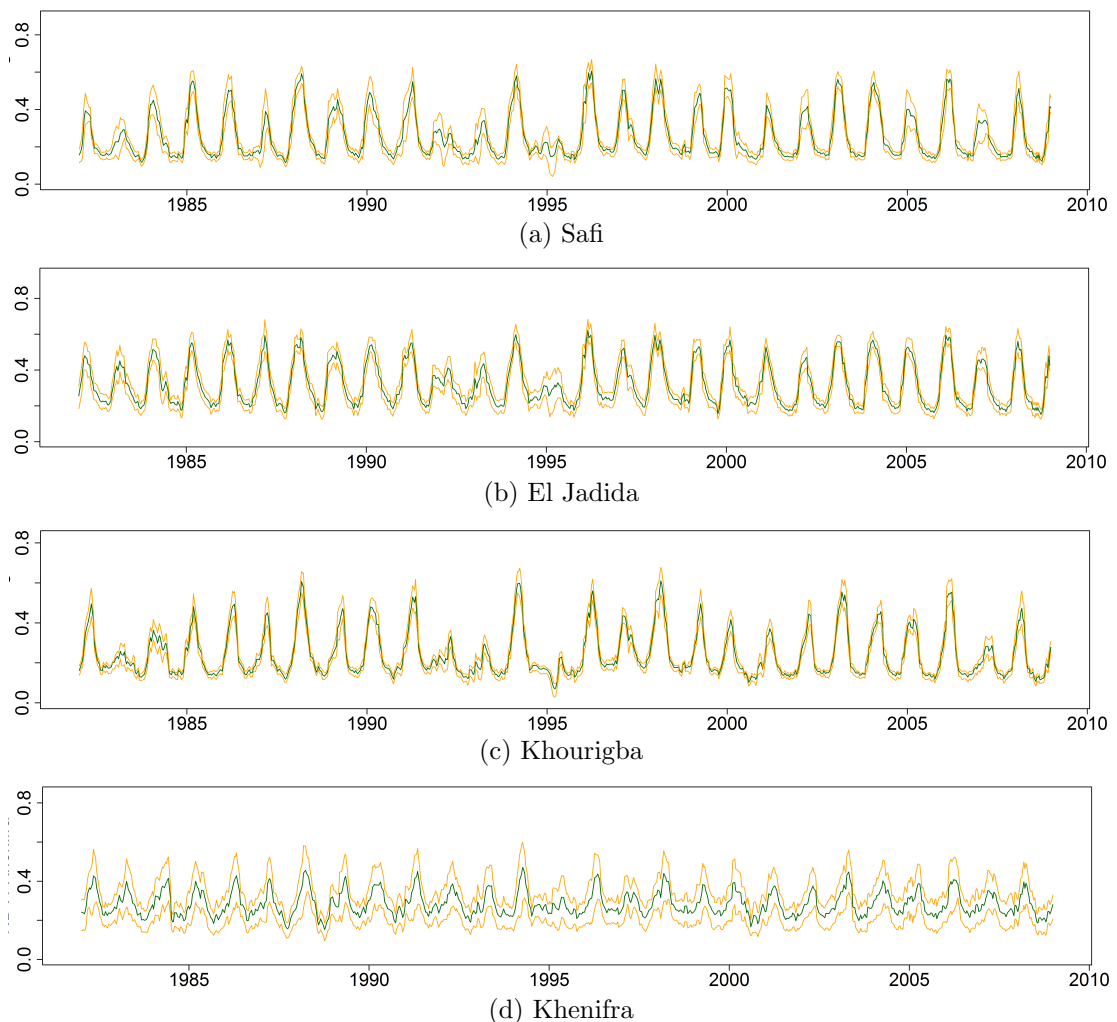
FIGURE 4.9 – Séries temporelles agrégées des quatre zones étudiées (Maroc) dont la localisation est présentée en Figure 4.8. Les premier et troisièmes quartiles sont également superposés.
