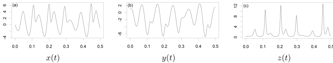
FIGURE 3.1 – Signal original du système Rössler-76 pour les variables x , y et z .
