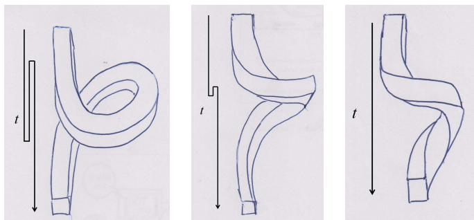
FIGURE C.2 – Différentes vues d'un mouvement de Reidemeister en 4D.
