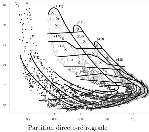
FIGURE 5.11 – Partition obtenue par la propagation directe-rétrograde systématique du domaine B_0 choisi dans la section de Poincaré.
