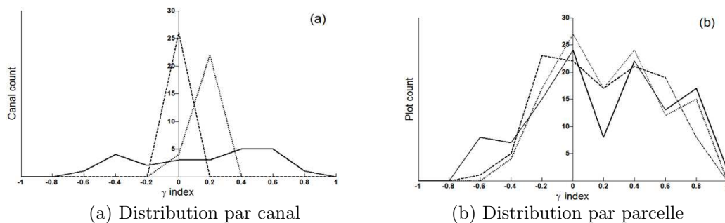
FIGURE 1.15 – Distribution de l'indice de priorité d'irrigation avant et après optimisation. Belaqziz S., Mangiarotti S. et al. [2].
