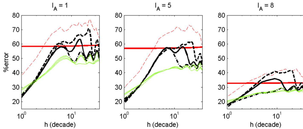
FIGURE 1.13 – Erreur de prévision (en %) présentée en fonction de l'horizon de prévision h : (a) pour les données non agrégées ( I_A = 1 ), puis (b) pour les données agrégées à I_A = 5 et (c) I_A = 8 . Une représentation logarithmique de l'horizon de prévision a été choisie pour rendre le développement initial de l'erreur plus visible tout en permettant de suivre les comportements observés à horizons longs. Le trait gras rouge est obtenu à partir d'une simple climatologie et la ligne en pointillés rouges à partir d'un modèle statistique saisonnier. Les autres lignes sont obtenues grâce à l'approche prédictive présentée dans le présent paragraphe (§1.5.2) et correspondent à différentes dimensions de reconstruction : d_r = 2 (lignes pointillées), d_r = 3 (trait plein noir) et d_r = 4 (tirets-pointillés), d_r = 5 à 8 (autres lignes vertes).
