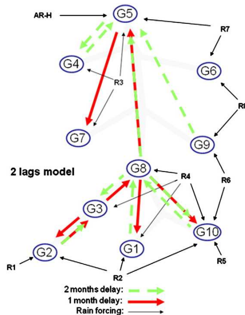
FIGURE 1.18 – Réseau des liens de causalité déduit des modèles « optimaux » obtenus après que certaines restrictions ont été identifiées. Les résultats sont présentés pour le modèle à double retard (flèches épaisses pleines pour les retards d'un mois et pointillées pour les retards de deux mois), les liens de forçage externes dues aux précipitations étant représentés par des flèches fines. Le lecteur est renvoyé à la publication originale pour une analyse détaillée de ce graphe [5].
