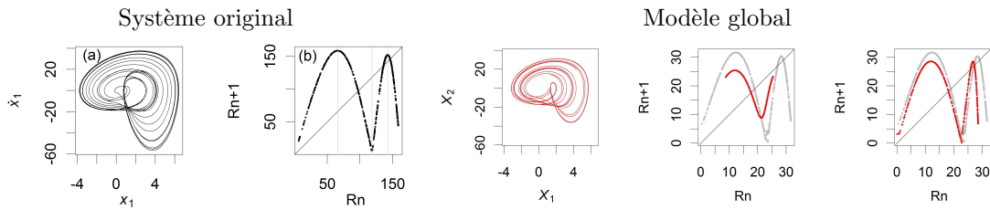
FIGURE 3.3 – Portraits de phase et applications de premier retour issus de la variable x du système Rössler (1 re et 2 e colonnes) puis issus du modèle global 10-termes (colonnes 3 à 5), la dernière applications de premier retour étant obtenue après l’ajustement manuel d’un paramètre.
