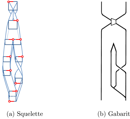
FIGURE 5.24 – Squelette (a) et gabarit (b) correspondant à la suspension (la plus simple possible) du système de Hénon.
