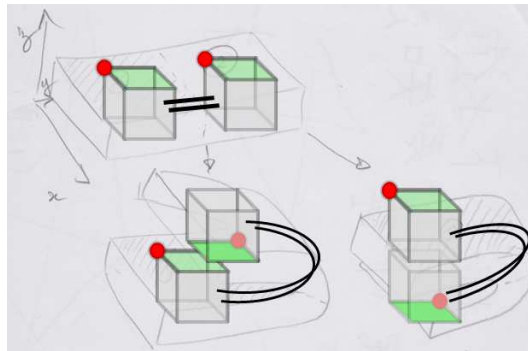
FIGURE 5.21 – plis d’une section 3D suivant (tx) pour des angles positif (à gauche) et négatif (à droite).
