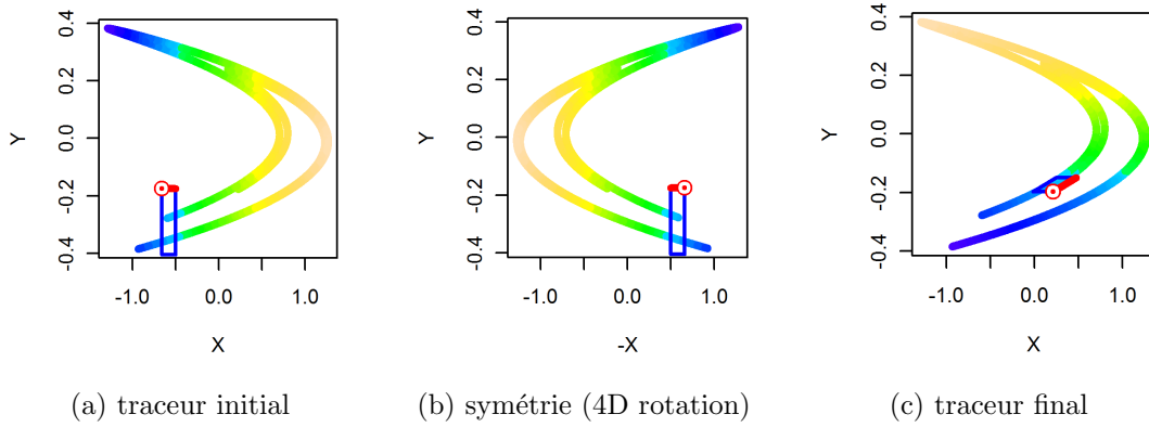
FIGURE 5.23 – Passage de l'état initial (a) au final (c) du traceur.
