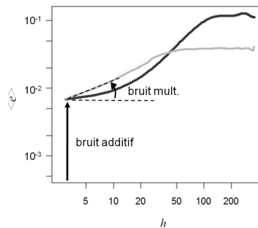
FIGURE 2.3 – Croissance de l'erreur RMS de prévision \langle e \rangle en fonction de l'horizon de prévision h : pour le modèle avec schéma d'assimilation (en noir), et pour l'approche par recherche d'états analogues dans l'espace des phases (en gris).
