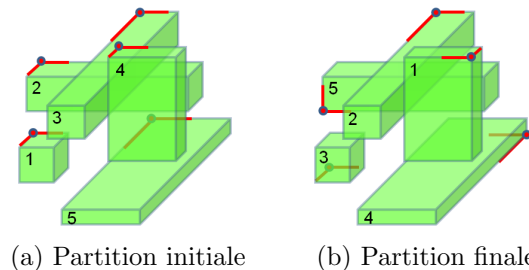
FIGURE 5.17 – Correspondance d'une section de Poincaré 3D à elle-même (exemple didactique).
