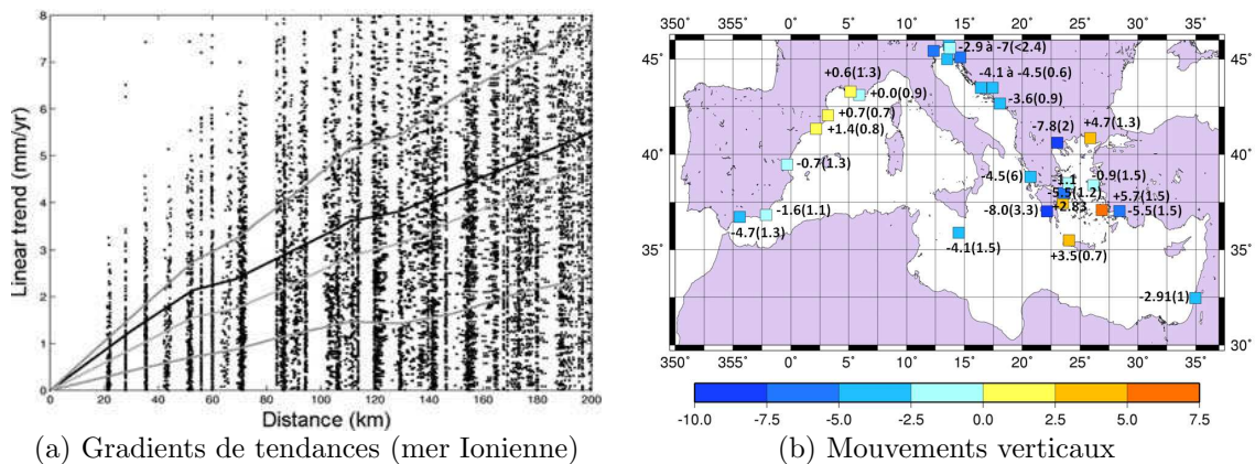
FIGURE 1.2 – (a) Différences des tendances linéaires du niveau de la mer (mm/an) en fonction de la distance entre points de mesures. (b) Mouvements verticaux de la croûte terrestre (et erreur associée) estimés par différences entre mesures altimétriques et marégraphiques (mm/an).
