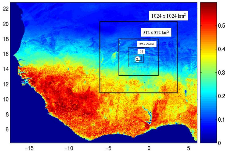
FIGURE 1.7 – Valeurs moyennes des séries temporelles normalisées NDVI AVHRR à 8 \times 8 \text{ km}^2 de résolution calculée sur la période 1982-2004 sur l’Afrique de l’Ouest. Les fenêtres avec des indices d’agrégation I_A = 8 à I_A = 6 centrées sur le site d’Agoufou dans le Sahel (région du Gourma, Mali) sont représentées. Le trait le plus saillant de cette carte est le gradient nord-sud du signal NDVI qui correspond à la distribution zonale des principaux types de végétation d’Afrique de l’Ouest.
