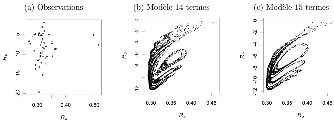
FIGURE 4.6 – Sections de Poincaré issues du jeu d'observation et des deux attracteurs obtenus à partir des modèles globaux à 14 et à 15 termes (Eqs. 4.2 et 4.3).
