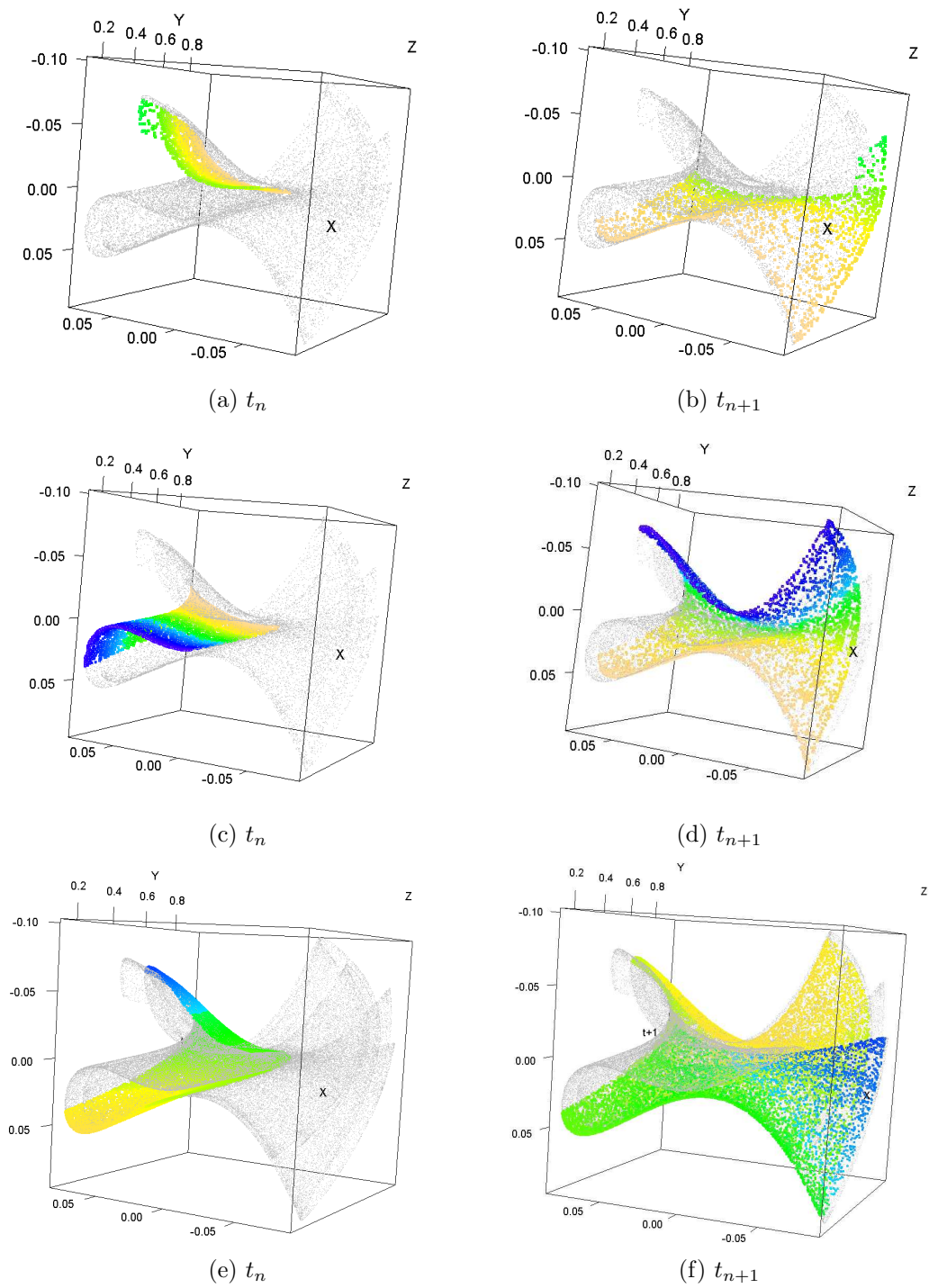
FIGURE 5.27 – Sections de l'attracteur 3D-Walking Stick [255] avec trois zones sélectionnées au temps t_n (à gauche) et propagation de cette zone sur l'attracteur au temps t_{n+1} .
