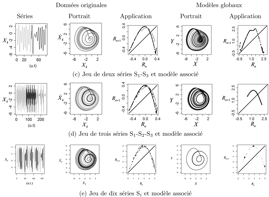
FIGURE 3.11 – Modèles globaux obtenus à partir de série temporelles analysées en association et produites par des ensembles de systèmes de Rössler indépendants. En première colonne sont présentées les séries temporelles concaténées (les différents niveaux de gris correspondent aux différents systèmes). Les portraits de phase et les applications de premier retour correspondants sont respectivement présentés dans les deuxième et troisième colonnes. Les portraits de phase et les application de premier retour produits par les modèles globaux sont tracés en quatrième et cinquième colonnes. Trois cas sont présentés relatifs à 2, 3 et 10 séries. Pour ce dernier cas, deux applications de premier retour sont présentées, le cas présentant un chaos plus développé a été obtenu en ajustant l'un des paramètres du modèle.
