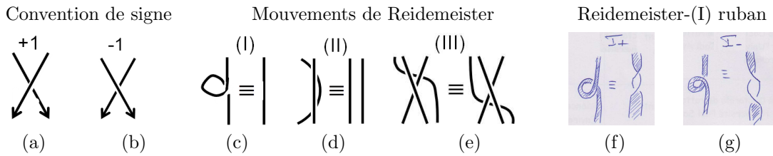
FIGURE 5.1 – Convention de signe de croisement et mouvements de Reidemeister de cordes et de rubans.
