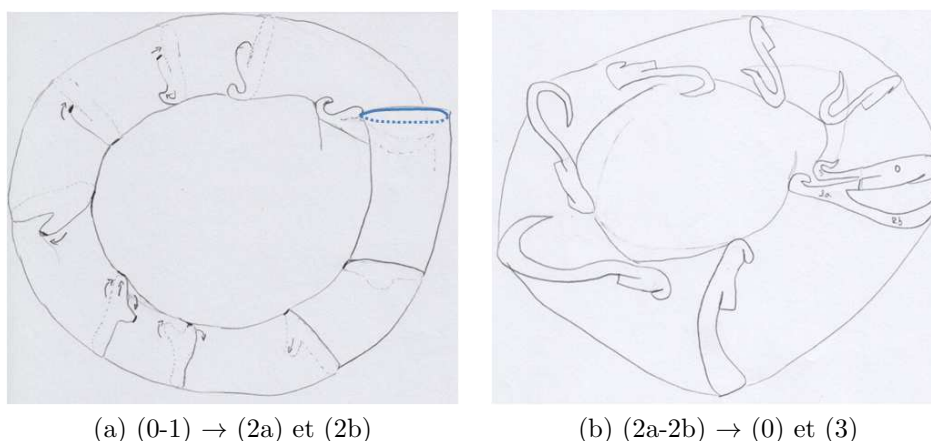
FIGURE 5.7 – Structure permettant l'auto-correspondance de la partition de la section de Poincaré présentée Fig. 5.6 vers elle-même.
