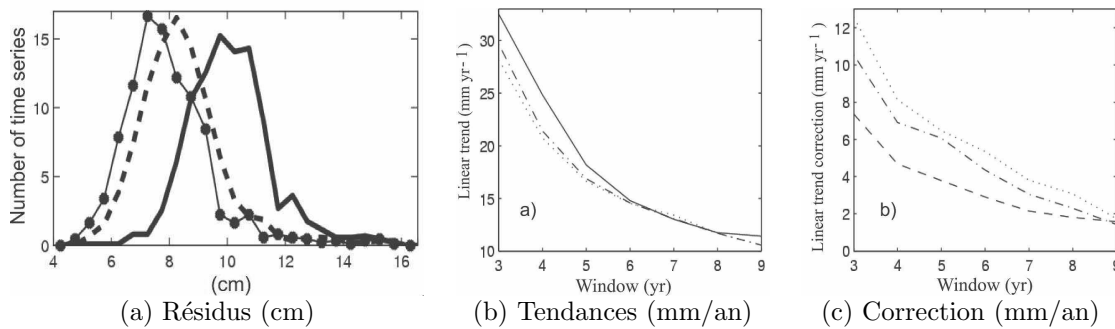
FIGURE 1.4 – (a) Variance (en cm) du signal marégraphique sans correction de charge atmosphérique (trait plein), après correction IB (tirets) et après correction du modèle barotrope MOG2D (points noirs); (b) Moyenne des tendances linéaires maximales (mm.yr an ) du niveau de la Mer Méditerranée en fonction de la taille des fenêtres considérées sans correction de charge (trait plein), avec correction IB (tirets-pointillés), avec correction barotrope MOG2D (pointillés); (c) Correction de tendance linéaires (mm.yr an ) résultant de la correction IB (tirets-pointillés), de la correction barotrope MOG2D (pointillés) et du passage de la correction IB à la correction MOG2D (tirets).
