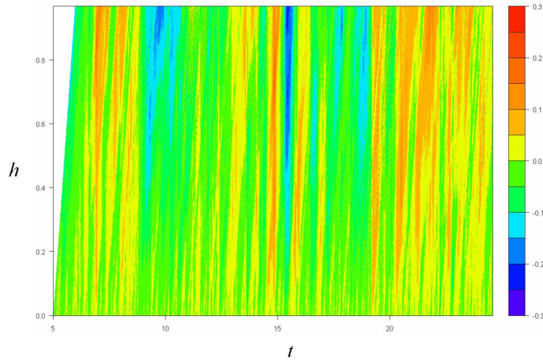
FIGURE 2.2 – Exemple de carte d’erreur de prévision e(t, h) en fonction du temps t et de l’horizon de prévision h obtenue ici pour le système de Lorenz-84 en utilisant un schéma d’assimilation de données de type ExKF.
