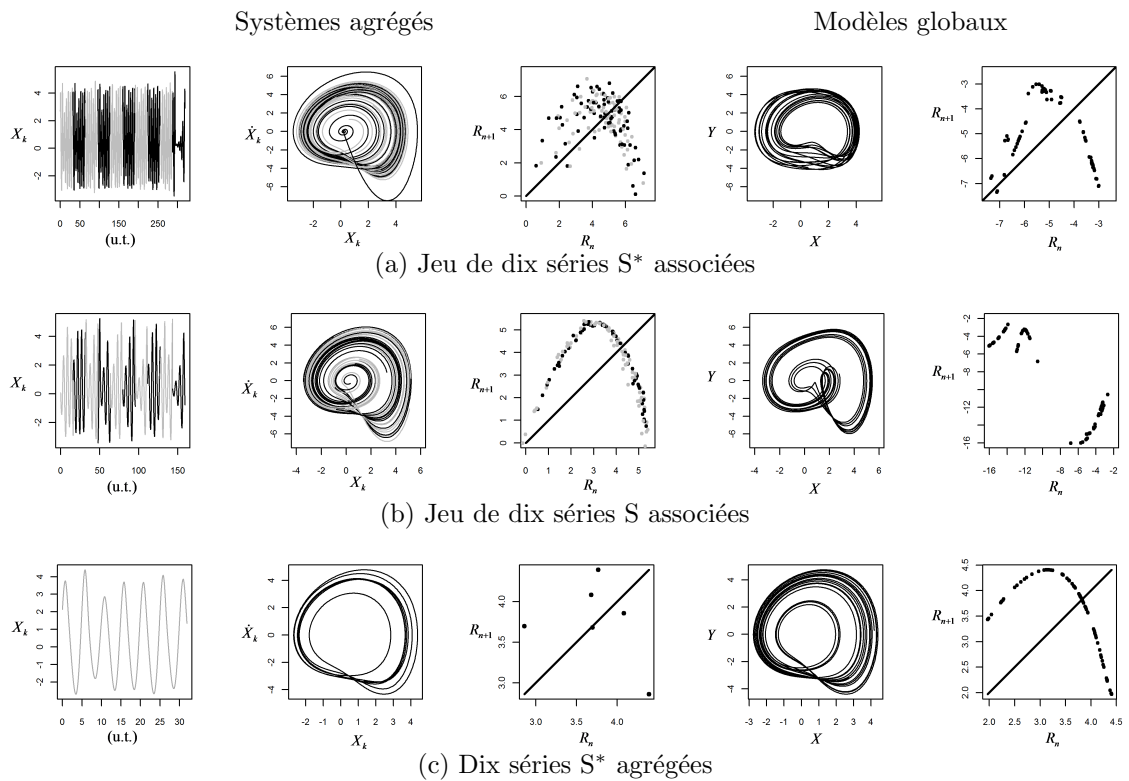
FIGURE 3.15 – Séries temporelles d'entrée (première colonne). Portraits de phase et applications de premier retour des séries temporelles agrégées à partir de systèmes de Rössler indépendants (colonnes 2 et 3) et produits par les modèles correspondants (colonnes 4 et 5).
