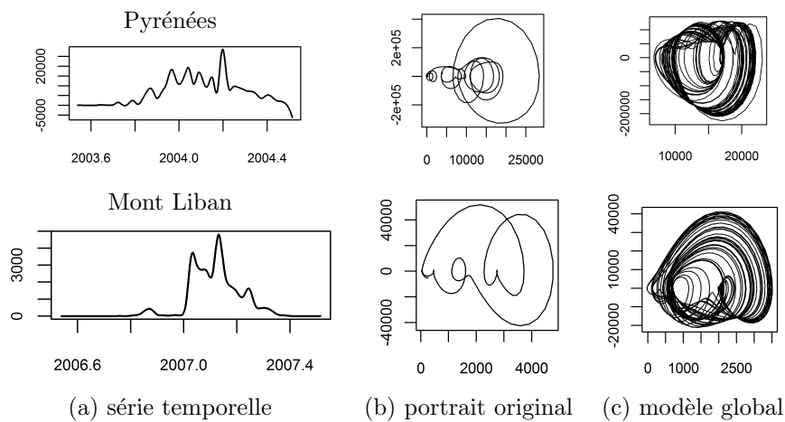
FIGURE 4.14 – Série temporelle d’une saison (à gauche), portrait de phase des données (au centre), puis du modèle (à droite). Les Pyrénées, année 2003-2004 (en haut), Le Mont Liban, année 2006-2007 (en bas).
