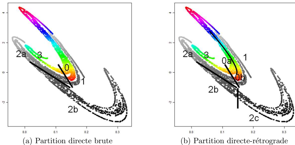
FIGURE 5.6 – Premières partitions (brute et améliorée) de la section de Poincaré.
