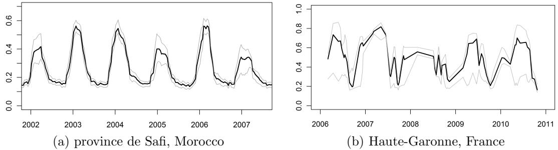
FIGURE 3.7 – Séries temporelles de l'indice de végétation NDVI observées depuis l'espace : (a) agrégées sur la province de Safi (Maroc) en faisant la moyenne spatialisée des mesures AVHRR (le produit développé par le GIMMS [285] a été utilisé à cette fin), et (b) agrégées à 320 m de résolution sur des parcelles situées à la latitude 43^{\circ}31'55'' de latitude et 1^{\circ}10'4'' en Haute-Garonne, dans le sud de la France (le produit d'origine à 8 m de résolution issue de FORMOSAT-2, une ortho-rectification et une correction des perturbations nuageuses ont été appliquées [150]).
