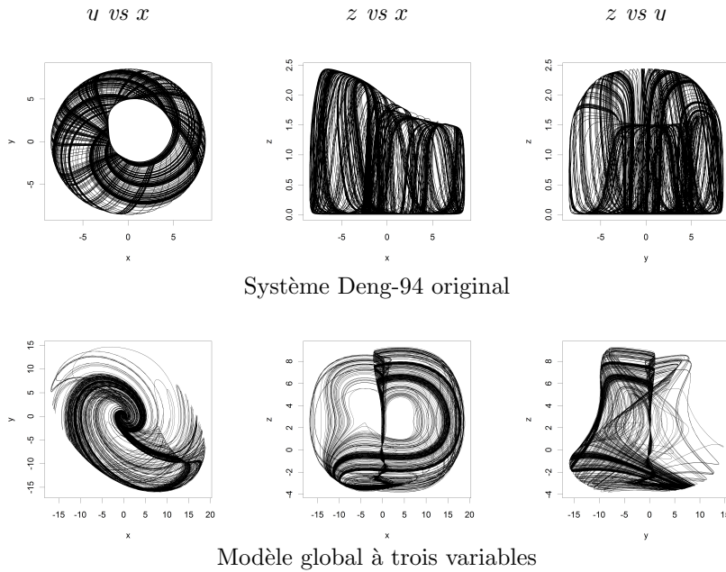
FIGURE 3.18 – Portraits de phase de l'attracteur original du système de Deng-94 (Eq. 3.20) (en haut) et d'un modèle à 9 paramètres obtenu à partir d'une solution périodique de Deng-94 (en bas).
