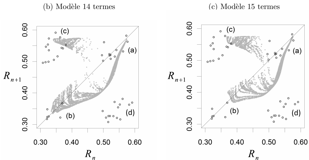
FIGURE 4.7 – Applications de premier retour des modèles 14 (à gauche) et 15-termes (à droite). L'application issue des données y est également superposée (petits ronds noirs).
