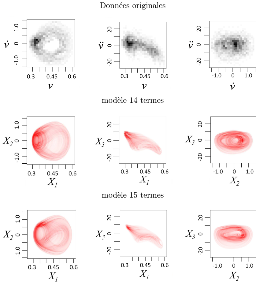
FIGURE 4.4 – Portraits de phase en densité (mêmes présentation que Fig. 4.2).
