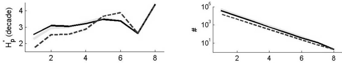
FIGURE 1.10 – Moyennes spatiales de l’horizon de prévisibilité H_P , et nombre de séries temporelles utilisées pour cette estimation, en fonction de l’indice d’agrégation spatiale I_A correspondant à 2^{2I_A-2} fois la résolution initiale de 8 \times 8 \text{ km}^2 . Les estimations présentées ont été estimées pour trois valeurs différentes de la dimension de plongement : d_e = 3 , d_e = 4 et d_e = 5
