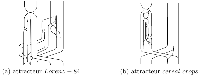
FIGURE 5.15 – Gabarits obtenus (a) pour l'attracteur de Lorenz – 84, et (b) pour l'attracteur cereal crops .
