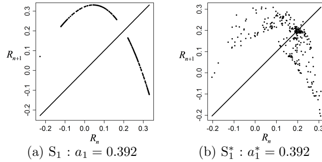
FIGURE 3.8 – Application de premier retour pour une section de Poincaré produites par un modèle indépendants S_k (a), et par les systèmes S_k^* en synchronisation de phase avec le système de Rössler de référence (b).
