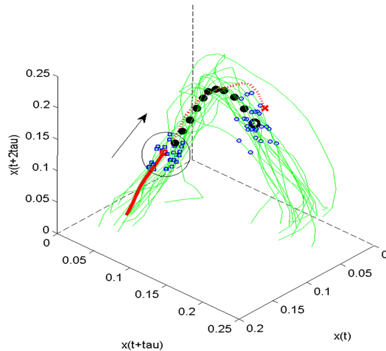
FIGURE 1.11 – La trajectoire géométrique de la série chronologique NDVI (voir Fig. 1.12) reconstruite dans un espace à 3 dimensions en utilisant les coordonnées retardées. La flèche noire indique la direction du flot (temps croissant). Les derniers états visités par le système sont représentés par une ligne rouge épaisse, le grand carré rouge correspond au dernier état visité par le système d'où sera lancée la prévision, et considéré comme l'état courant. La ligne en pointillés rouges représente la suite de la trajectoire dont on cherche à faire la prévision, mais que l'on a retirée ici pour analyser les capacités prévisionnelles de l'approche. Les états préalablement visités par le système dans le proche voisinage de l'état courant sont marqués par de petits carrés bleus. Le suivi de ces états voisins après un horizon h est représenté par de petits cercles bleus. La valeur réellement observée à l'horizon h et que l'on cherche à prévoir est indiquée par la croix épaisse rouge. La trajectoire de la prévision est délimitée par les grands points noirs. Les mêmes symboles correspondant à ces différents états sont utilisés dans la représentation temporelle (Fig. 1.12).
