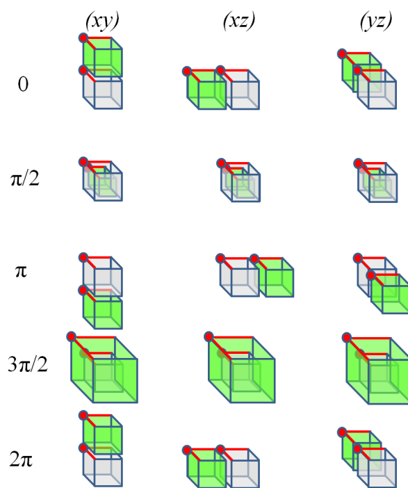
(b) Section 3D d'un flot 5D
