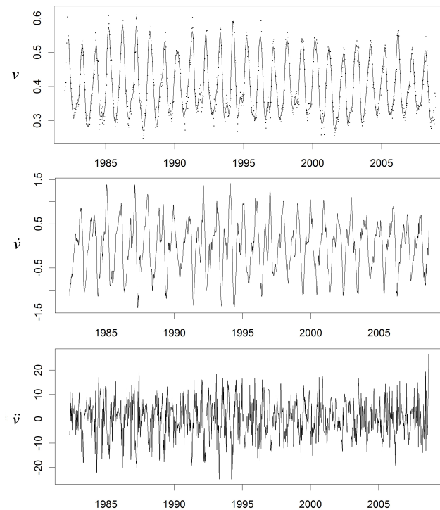
FIGURE 4.1 – Signal de l'indice NDVI de végétation moyenné \nu pour une zone d'étude située sur le Nord du Maroc. Le signal agrégé est présenté avant (points) et après lissage (trait plein). La première dérivée \dot{\nu} puis la seconde dérivées \ddot{\nu} sont données dans les panneaux suivants.
