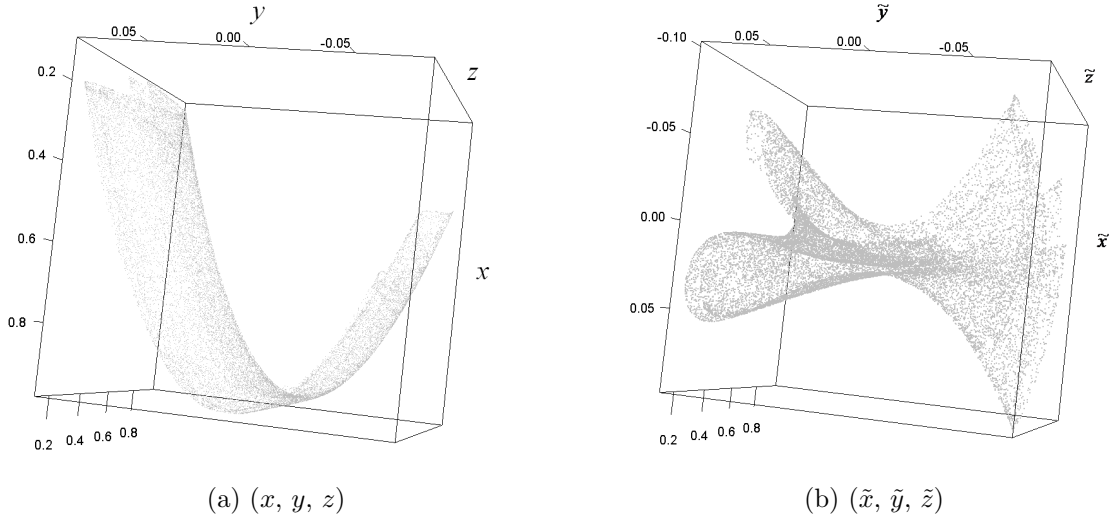
FIGURE 5.26 – Portrait original (a) et portrait anamorphosé suivant le difféomorphisme présenté en (5.29) (b) de l'application 3D walking stick (Eq. 5.28, [255]).
