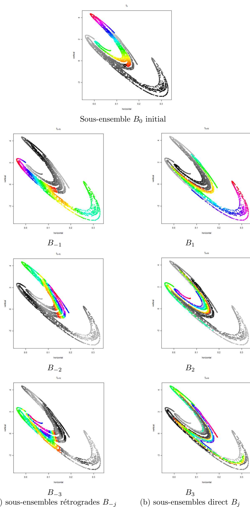
FIGURE 5.5 – Sections de Poincaré de l'attracteur de Lorenz-84 avec zone sélectionnée B_0 et propagation de cette zone sur l'attracteur suivant le sens direct B_i, i = 1..3 et rétrograde B_{-i}, i = 1..3 .
