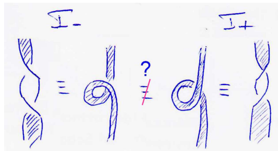
FIGURE C.1 – Premier mouvement de Reidemeister en dimension quatre, paradoxe de l'enroulement bidirectionnel.
