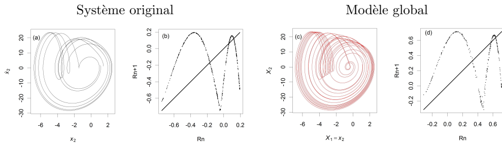
FIGURE 3.2 – Portraits de phase (colonne de gauche) et applications de premier retour (colonne de droite) issus de la série originale de la variable y du système Rössler (haut) du modèle global 9-termes (deuxième ligne) obtenu à partir de celle-ci.
