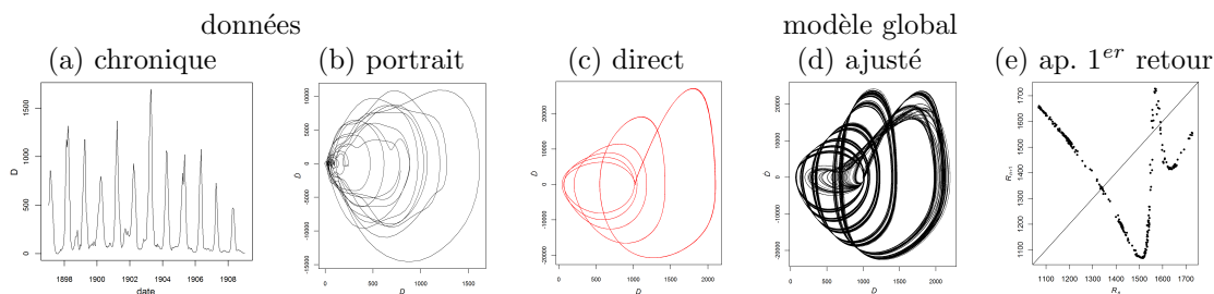
FIGURE 4.15 – Série temporelle du nombre de décès par semaine (a), portrait de phase des données (b), puis du modèle direct (c), puis du modèle ajusté (d). application de premier retour du modèle ajusté (e).
