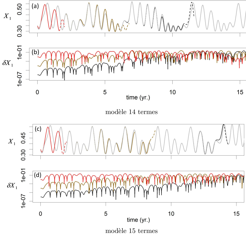
FIGURE 4.5 – Tests de sensibilité aux conditions initiales pour les modèles à 14 termes (a-b) et à 15 termes (c-d). Quatre simulations ont été effectuées pour chaque modèle. Les lignes grises dans (a) et (c) correspondent aux solutions de référence de X_1 en fonction du temps t (en année). Les autres trajectoires (lignes colorées) ont été obtenues en appliquant une petite perturbation de 10^{-2} , 10^{-4} et 10^{-6} sur les conditions initiales (sur X_1 uniquement). Les signaux de différence \delta X_1(t) à la trajectoire de référence sont présentés en (b) et (d).
