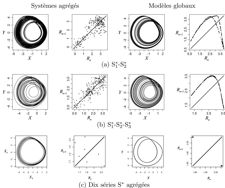
FIGURE 3.13 – Portraits de phase portraits et applications de premier retour issus des séries temporelles agrégées de systèmes en synchronisation de phase (colonne 1 et 2) et issus de modèles qui en ont été obtenus (colonnes 3 et 4).
