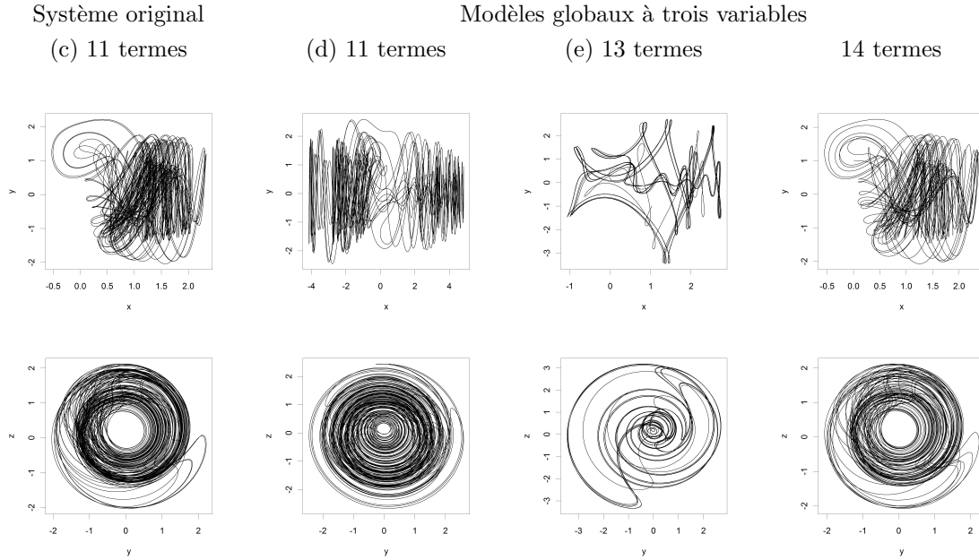
FIGURE 3.17 – Portraits de phase x vs y (ligne du haut) et y vs z (ligne du bas) de l'attracteur original du système de Lorenz-84 (Eq. 5.9) (gauche) et de trois modèles globaux de 11 (2 e colonne), 13 (3 e colonne) et 14 (4 e colonne) termes obtenus à l'aide de l'algorithme multivarié (cf. §2.3.3).
