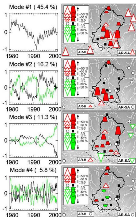
FIGURE 1.17 – Série chronologique normalisée (colonne de gauche) et répartition spatiale associée (colonne de droite) pour les quatre modes principaux de la décomposition en Fonction Empirique Orthogonale (classées de haut en bas par pourcentage décroissant de variance expliquée) résultant d'une analyse conjointe des données de pluies cumulées et de niveau des eaux souterraines. Le % de variance expliquée associé à chaque station est donnée sur la balance des panneaux de colonne de gauche, les triangles indiquent les stations de pluies et les trapèzes les stations de niveau d'eau souterraine.
