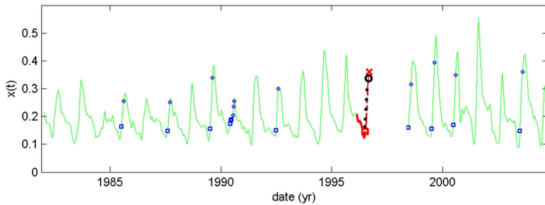
FIGURE 1.12 – La ligne verte représente le signal original informatif. Les derniers états visités par le signal sont représentés par la ligne épaisse rouge, jusqu’au dernier état d’où la prévision doit être lancée. Les petits cercles bleus correspondent aux états proches de l’état courant (voir Fig. 1.11). Les petits cercles bleus représentent l’évolution temporelle après un horizon h . Le cercle noir représente la prévision obtenue à partir des valeurs moyennes pondérées de l’évolution des états voisins (calculées dans l’espace des phases, voir Fig. 1.11). Cette prévision peut être comparée. L’observation est représentée par une croix rouge. Les points noirs représentent les prévisions intermédiaires, tandis que la ligne en pointillés rouge correspond aux états intermédiaires observés qui ont été temporairement retirés pour tester les capacités prévisionnelles de l’approche.
