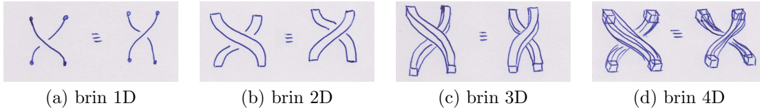
FIGURE 5.16 – En dimension quatre, le croisement de brins indépendants n'est qu'apparent, qu'il s'agisse de brins constitués de simples lignes (a), de surfaces (b) de volumes (c) ou d'hypervolumes (d).
