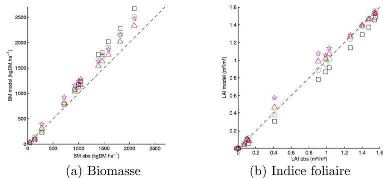
FIGURE 1.14 – Relation entre variables estimées, biomasse (a) et indice foliaire (b), en fonction de la valeur "observée" (générée artificiellement). Les symboles renvoient à différents modes d'inversion basés sur les données de rétrodiffusion (□), les indices NDVI (△), ou les deux combinés lors d'une optimisation mono- (☆) ou bi-objectif (○).
