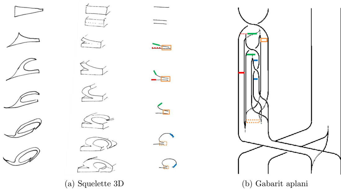
FIGURE 5.13 – (a) Passade d’une représentation 3D à une représentation 2D permettant de faire émerger une branche et de fournir une représentation plane du branchement entre les différents sous-ensembles de la section de Poincaré. (b) Gabarit ainsi obtenu. Le code de couleur permet de visualiser la zone d’émergence au sein du gabarit.
