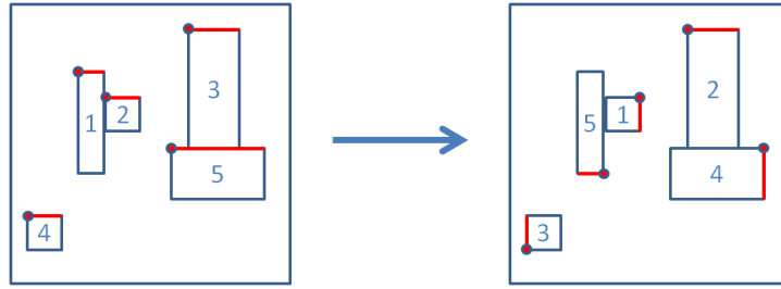
FIGURE 5.3 – Schéma d'exemple d'application d'une section de Poincaré vers elle-même visant à construire une matrice de rotation de premier retour.
