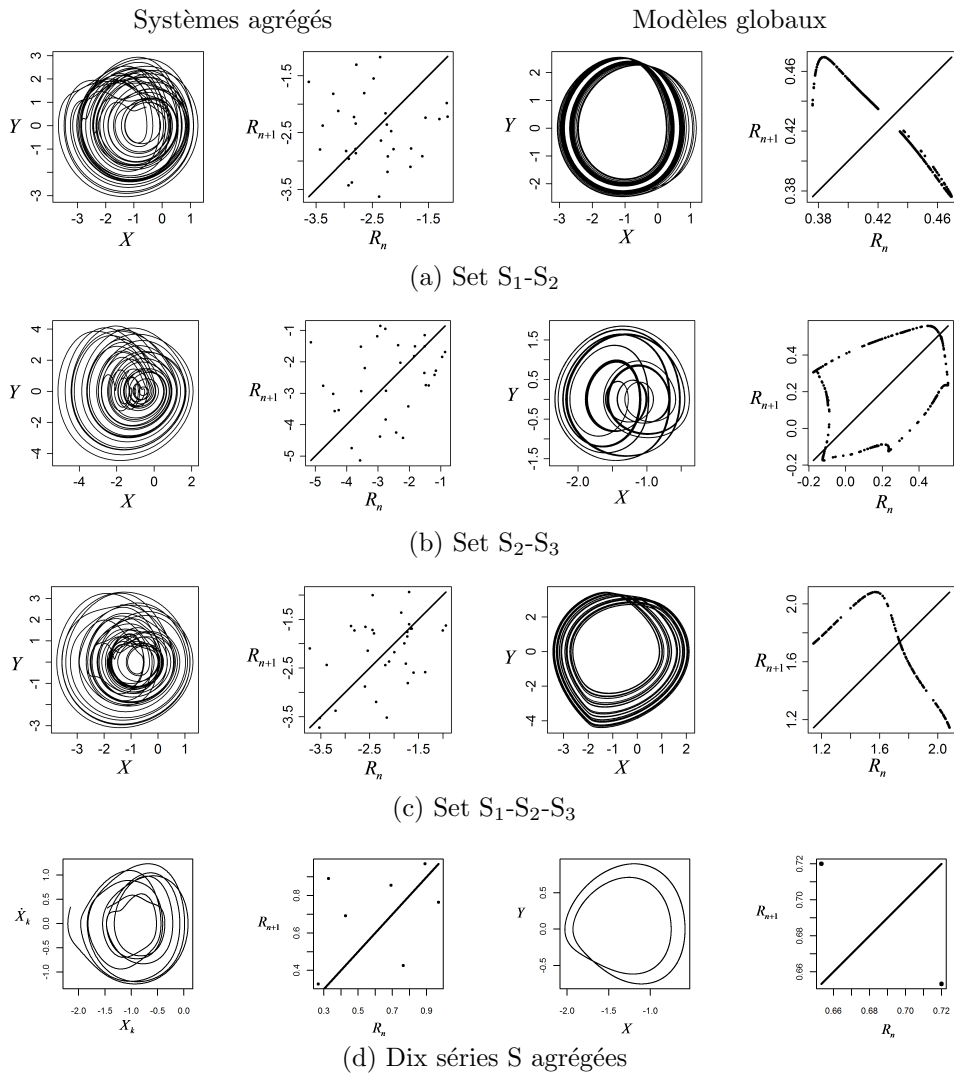
FIGURE 3.14 – Portraits de phase et applications de premier retour des séries temporelles agrégées à partir de systèmes de Rössler indépendants (colonnes 1 et 2) et produits par les modèles correspondants (colonnes 3 et 4).
