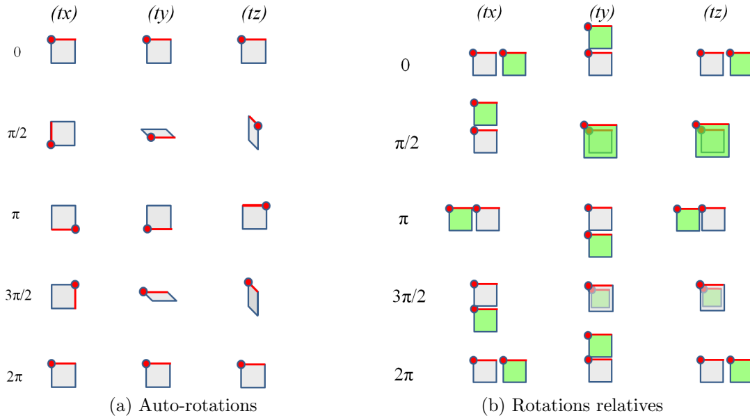
FIGURE 5.22 – Mouvements de rotation possibles pour un flot dans \mathbb{R}^4 présentant un ensemble de Poincaré 2D.
