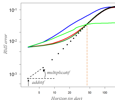
FIGURE 4.3 – Croissance de l'erreur de prédiction en fonction de l'horizon de prévision h pour le modèle associé à différents types de schéma d'assimilation de données : filtre de Kalman étendu (bleu), filtre de Kalman d'ensemble (rouge, [118]), synchronisation directe et rétrograde (vert foncé, [67]). Une méthode de simple réinitialisation a également été utilisée (pointillés). Ces résultats sont à comparer à la prévision basée sur le suivi de trajectoires analogues dans l'espace des phases qui ne nécessite pas de modèle dynamique (vert clair). Pour permettre la comparaison, le niveau de bruit additif associé aux prévisions avec schéma d'assimilation a été ajusté manuellement sur celui de la méthode sans modèle. Les modèles associés aux schémas d'assimilation de données les plus performants [67, 118] permettent de diminuer très significativement la vitesse de croissance du bruit.
