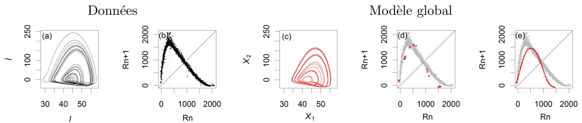
FIGURE 3.6 – Portraits de phase (colonne de gauche) et applications de premier retour (colonnes centrale et de droite) issus l'intensité de courant I(t) mesurée à partir de l'expérience présentée en paragraphe 3.3 et des deux modèles globaux de 21 termes obtenus de ce jeu de données en utilisant une deux fenêtres de tailles différentes (cf. Fig. 3.5) : le premier est issu d'une fenêtre courte (deuxième ligne), le second d'une fenêtre plus longue (troisième ligne). Les applications de premiers retour issus des modèles obtenus directement par l'algorithme GloMo sont tracées en colonne centrale. Un modèle supplémentaire obtenu après ajustement de paramètre est tracés en colonne de droite.
