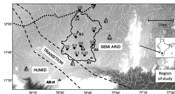
FIGURE 1.16 – Carte présentant l’emplacement géographique des stations pluviométriques (R1 à R9) et les postes de niveau des eaux souterraines (G1 à G10). AR-H et AR-SA sont les centres de la grille de données de pluie moyennes (voir texte) dans les zones climatiques humides et semi-arides, respectivement. La ligne noire indique la limite de la sous-bassin Gundal et les lignes blanches des différents cours d’eau et leurs affluents. L’échelle de gris est révélateur de la topographie (altitude en blanc).
