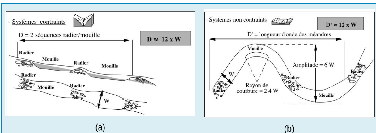
Figure 1 : Illustration de la succession des séquences de faciès « radier/mouille » pour des cours d'eaux évoluant (a) dans des lits contraints par la roche mère, et (b) dans des vallées alluviales à substrat meuble (Circulaire DCE 2007/22 du 11 avril 2007)
