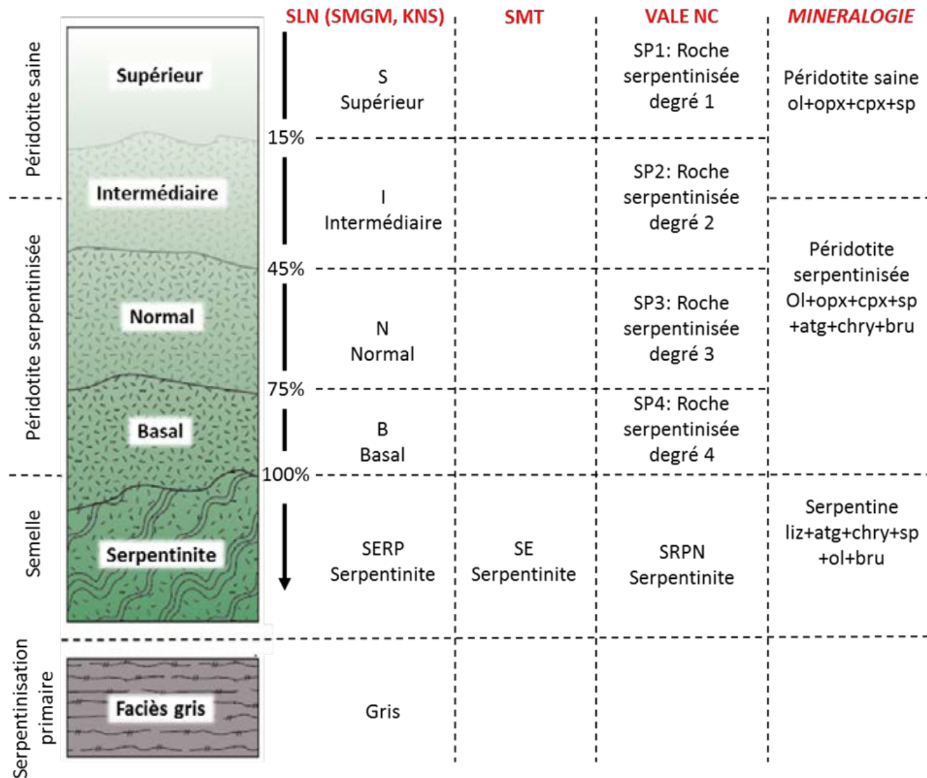
Figure 5 : Serpentinisation des péridotites. Terminologie comparée du degré de serpentinisation des péridotites par les différents acteurs miniers. Ol : olivine, opx : orthopyroxène, cpx : clinopyroxène, sp : spinelle, atg : antigorite, chry : chrysotile, bru : brucite, liz : lizardite.
