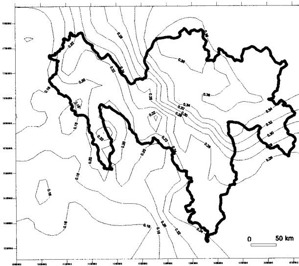
Figure 4 Isohyètes interannuelles et localisation des postes pluviométriques dans le bassin Nazas-Aguanaval et ses environs. Interannual isohyets and location of rain gauges in the Nazas-Aguanaval basin and surrounding areas.
