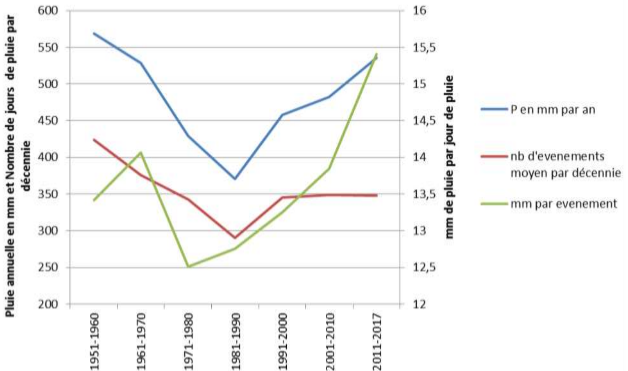
Figure 11 : évolution de la pluie annuelle (moyenne par décennie), du nombre de jours de pluie (par décennie) et de la moyenne de la pluie tombée par jour de pluie, dans le Bassin du Niger Moyen, 1951-2017
