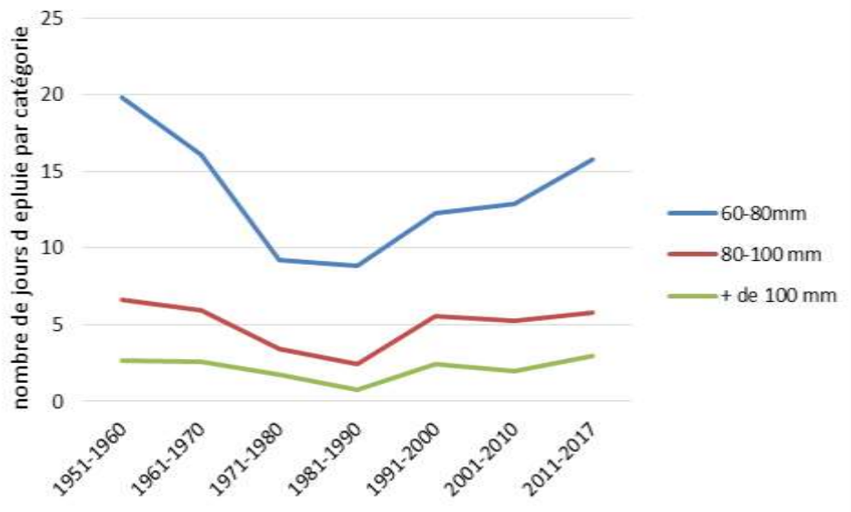
Figure 13 : évolution par décennie du nombre de jours de pluie de plus de 60, 80 et 100 mm en 24h, Sénégal, par décennie, de 1951 à 2017
