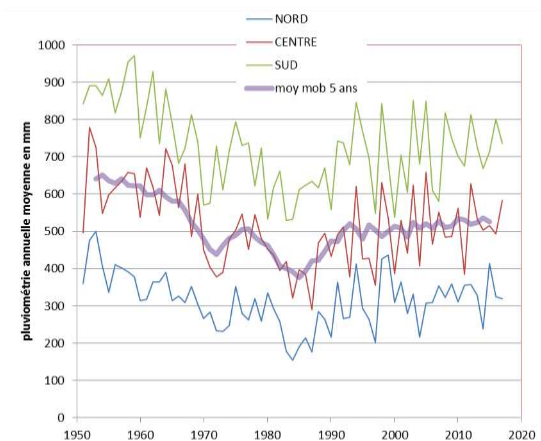
Figure 8 : évolution de la pluviométrie moyenne dans le bassin Moyen du Niger de 1951 à 2017
