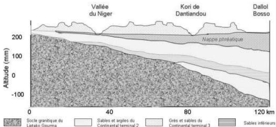
Figure 1 : configuration de la nappe du CT3, affleurante ou proche de l’affleurement dans les bas-fonds et les vallées les plus profondes à l’ouest du bassin sédimentaire des Iullemeden (d’après Montfort 1996, in Favreau, 2000)
