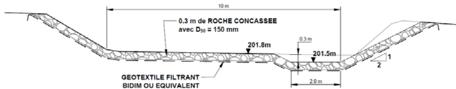
Figure 21 : Exemples de stations limnimétriques selon l'importance du creek (source Golder)
