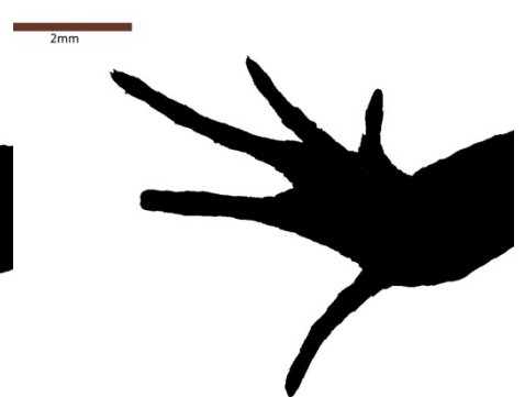
Caledoniscincus auratus
