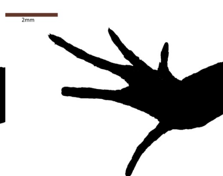
Caledoniscincus auratus
