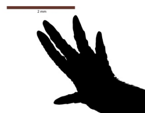
Nanoscincus mariei
