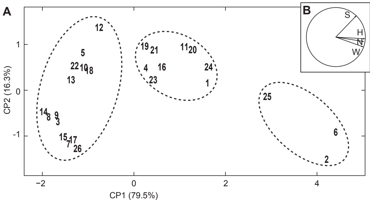
Figure 3. A. Plan principal d'une analyse en composantes principales (ACP) montrant les groupements d'îlots en fonction de quatre facteurs ( N , S , H , W ). L'ACP a été réalisée à l'aide de FACTOMINER (Lê, Josse & Husson 2008) sous R (R-core Team 2018). Les ellipses ont été définies à l'aide de l'algorithme de classification hiérarchique de FACTOMINER. Voir la Figure 1 pour la numérotation des îlots. B. Cercle des corrélations.
