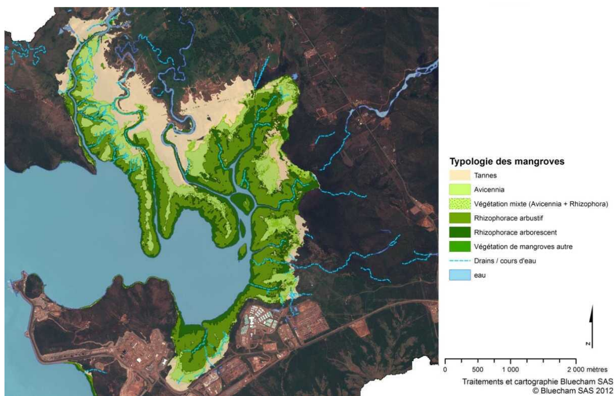
Figure 24 : Typologie des mangroves, Anse de Vavouto en Novembre 2010
