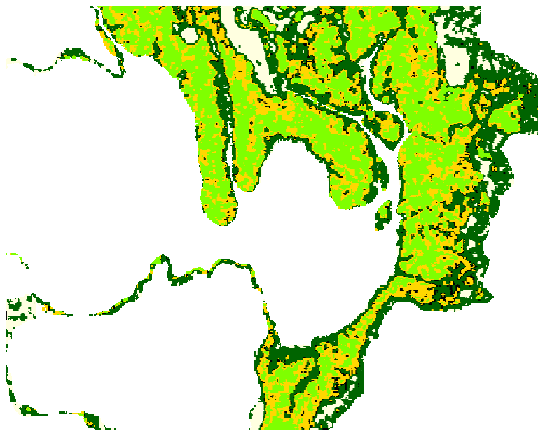
Figure 48 : Classification obtenue à partir de l'image radar du 9 décembre 2011
