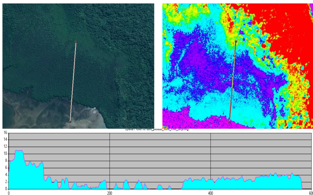
Figure 54: Image Pléiade tri-stéréoscopique du 13/07/2012 sur la mangrove de la Kwé Binyi (en haut à gauche); modèle numérique de surface dérivé des données tri-stéréoscopiques Pléiade du 13/07/2012 (à droite); Profil du nord au sud des altitudes de la canopée de la mangrove de la Kwé Binyi (en bas) - traitements Bluecham SAS et SERTIT (Université de Strasbourg), © CNES 2012, Distribution Astrium Services / Spot Image S.A., France, tous droits réservés. Usage commercial interdit.
