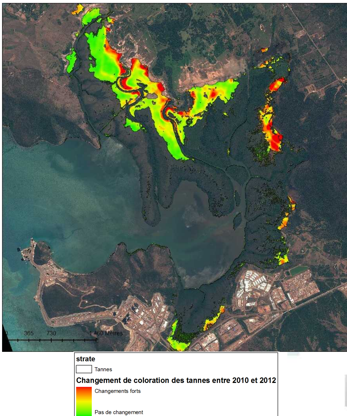
Figure 42: Variations spatiales de la rougeur des tannes entre novembre 2010 et juin 2012.
