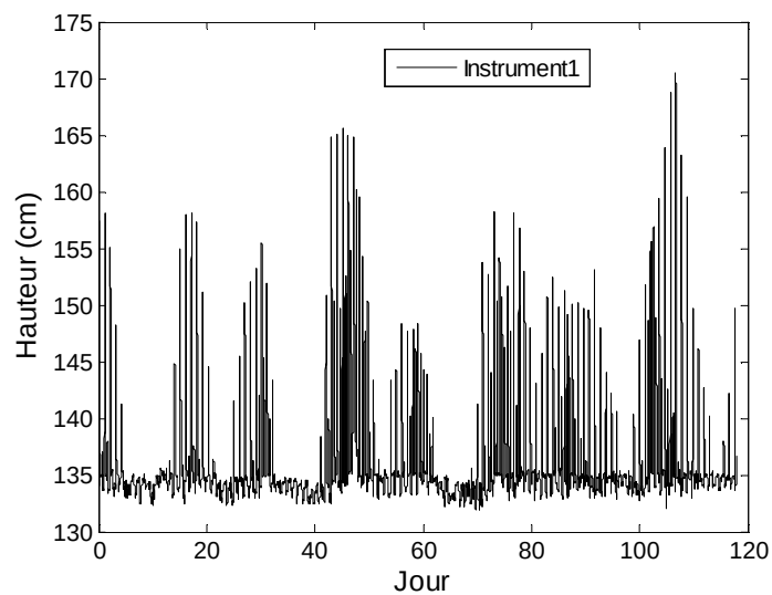
Figure 42 : marégramme sur 3 mois - Instrument 1
