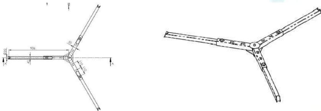
Figure 18 : Schémas du gabarit de montage
