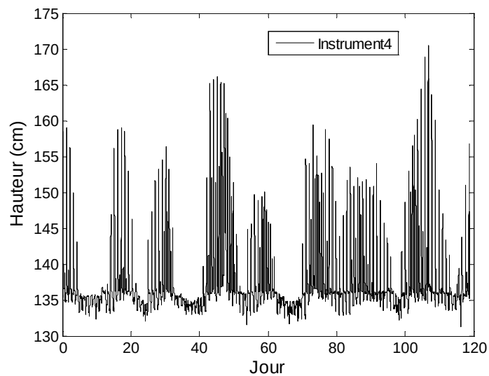
Figure 43 : marégramme sur 3 mois - Instrument 4
