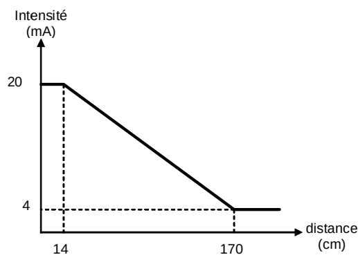
Figure 8 : Conversion Intensité - Distance
