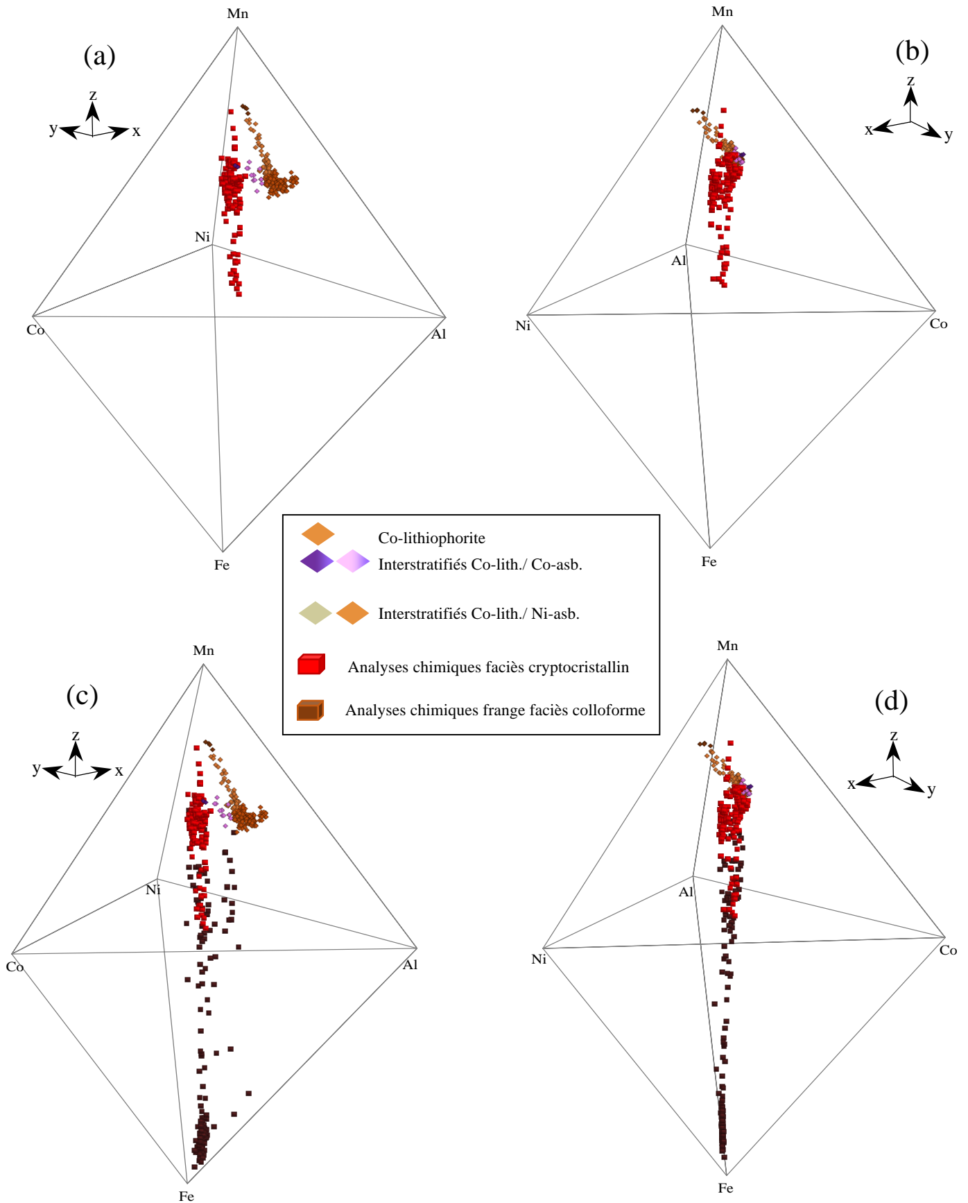
Figure 24 : Projection dans un diagramme à 5 dimensions Fe-Al-Mn-Ni-Co des analyses obtenues à la microsonde électronique sur les oxydes de manganèse à faciès colloforme et cryptocristallin des sites du Koniambo et de Goro.
