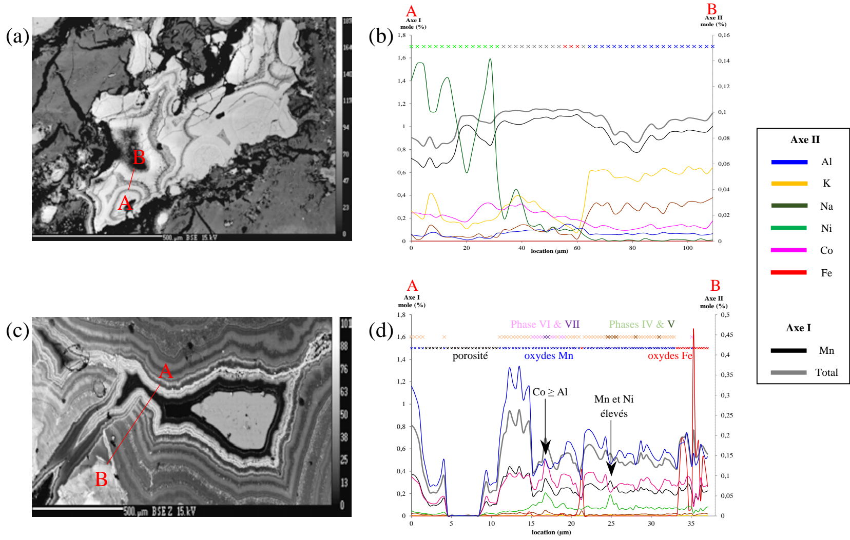
Figure 5 : Images MEB (mode électrons rétrodiffusés) illustrant l'organisation structurale des oxydes de manganèse dans les fractures de la latérite de transition (a) du massif du Koniambo et (c) du site de Goro.
