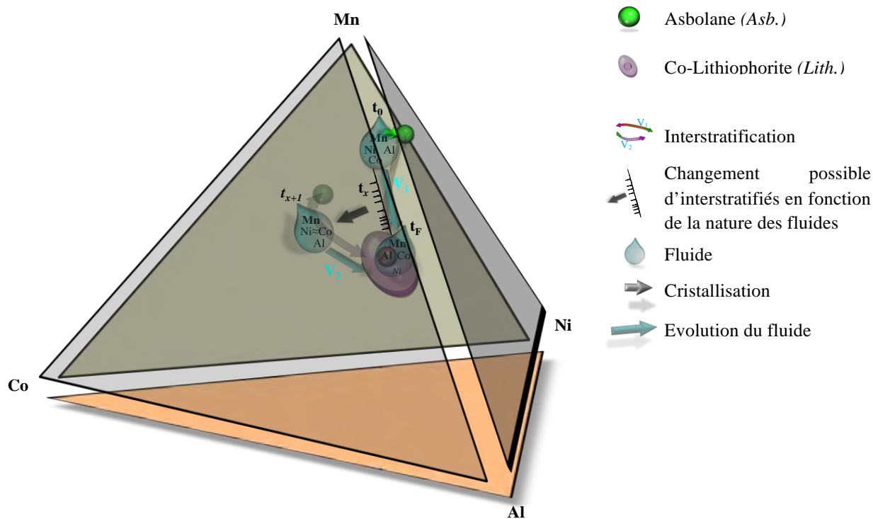
Figure 18 : Modèle d'évolution dans un diagramme 4 dimensions Al-Co-Ni-Mn d'un fluide permettant d'expliquer les successions de phyllomanganates observées dans les fractures des latérites de transition du site de Goro.
