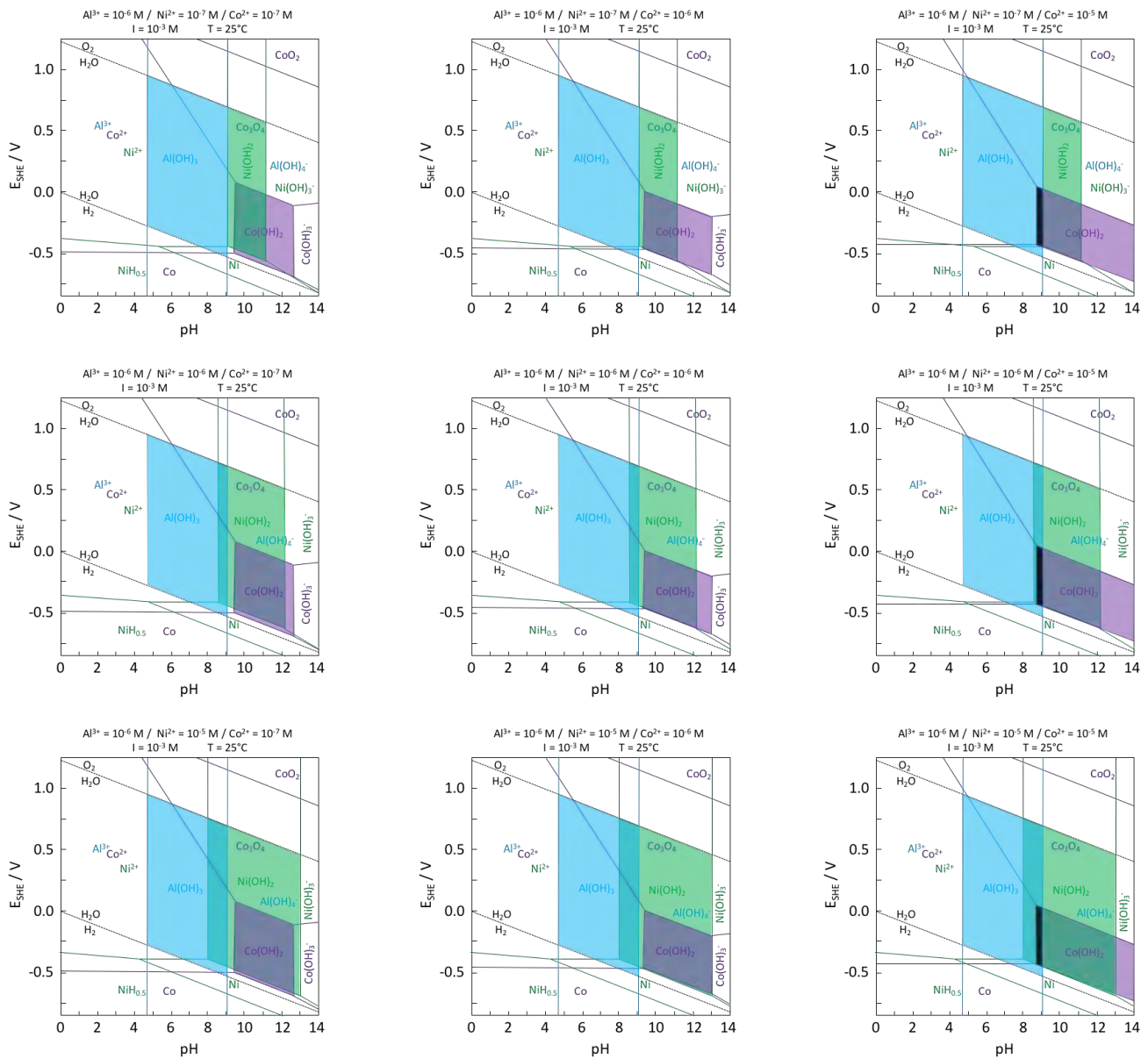
Figure 33 : Superposition des diagrammes de Pourbaix ( P_{atm} , 25°C) illustrant les zones de recouvrement éventuel des domaines de stabilité de Al(OH)_3 , Ni(OH)_2 et Co(OH)_2 (feuilletés élémentaires des interstratifiés asbolane/lithiophorite du site de Goro) pour différentes concentrations en ions Ni^{2+} et Co^{2+} en solution ( [Al^{3+}] = 10^{-6} mol/L). Pour des raisons de clarté, le diagramme de Pourbaix de MnO_2 n'est pas représenté.
