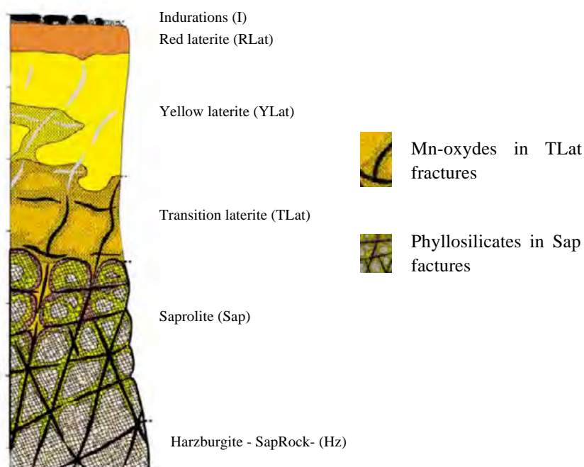
Figure 3 : Représentation schématique d'un profil type d'altération sur péridotites indiquant l'emplacement des minéralisations de type phyllosilicates et oxydes-Mn.
