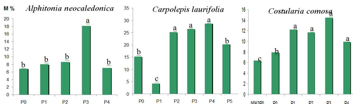
Figure 74 : Intensité de mycorhization (M en %) des 3 espèces testées, après 1 an de culture en pot, dans un sol ultramafique fertilisé avec des doses croissantes de P.
