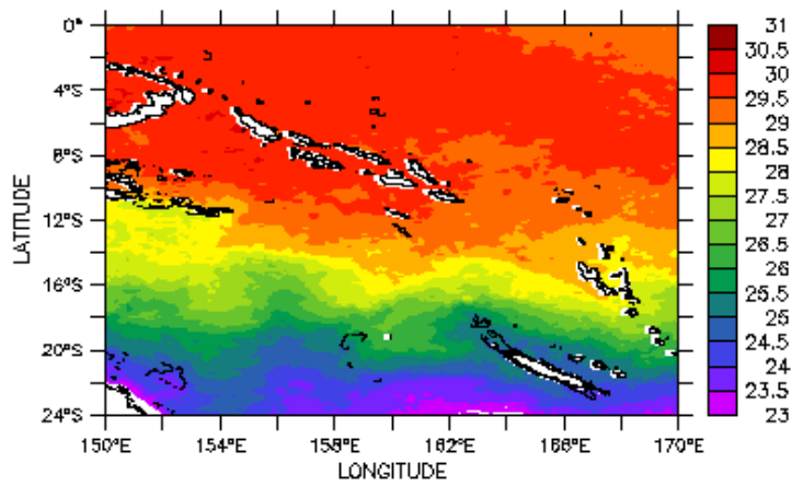
SST GRHSST
