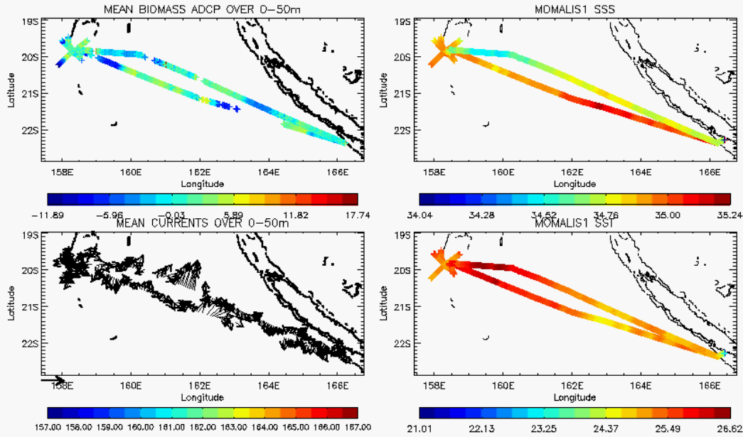
Fig. 19. Résumé des données in situ collectées durant les trajets de l' Alis ; la route au sud est l'aller. Haut, gauche scattering volume (SV, en dB) en anomalie sur toute la période (on retire la moyenne sur toute la période) ; les valeurs les plus fortes sont positives et les moins fortes sont négatives. Haut, droite : données de salinité de surface. Bas, gauche : courants moyens sur 50 m ; la longueur de la flèche en mage de la figure indique 0.5 m/s. Bas, droite : température de surface.
