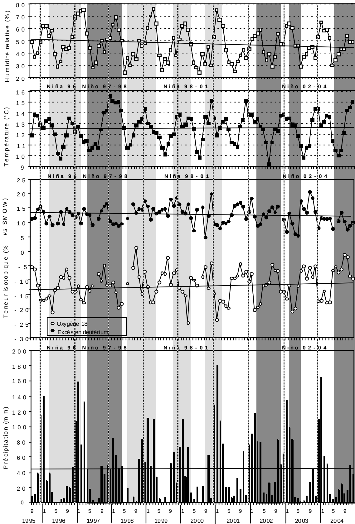
Fig. 3 Données mensuelles, à la station de Laica Cota entre 1995 et 2004, des teneurs en Humidité relative, Température, Oxygène 18, Excès en deutérium, et hauteur des pluies. Durant la période d'étude, les phases modérées à fortes La Niña et El Niño (valeurs S.O.I.) sont symbolisées en gris clair et gris foncé, respectivement. Pour les intensités de ces phases se reporter à la figure 7.
