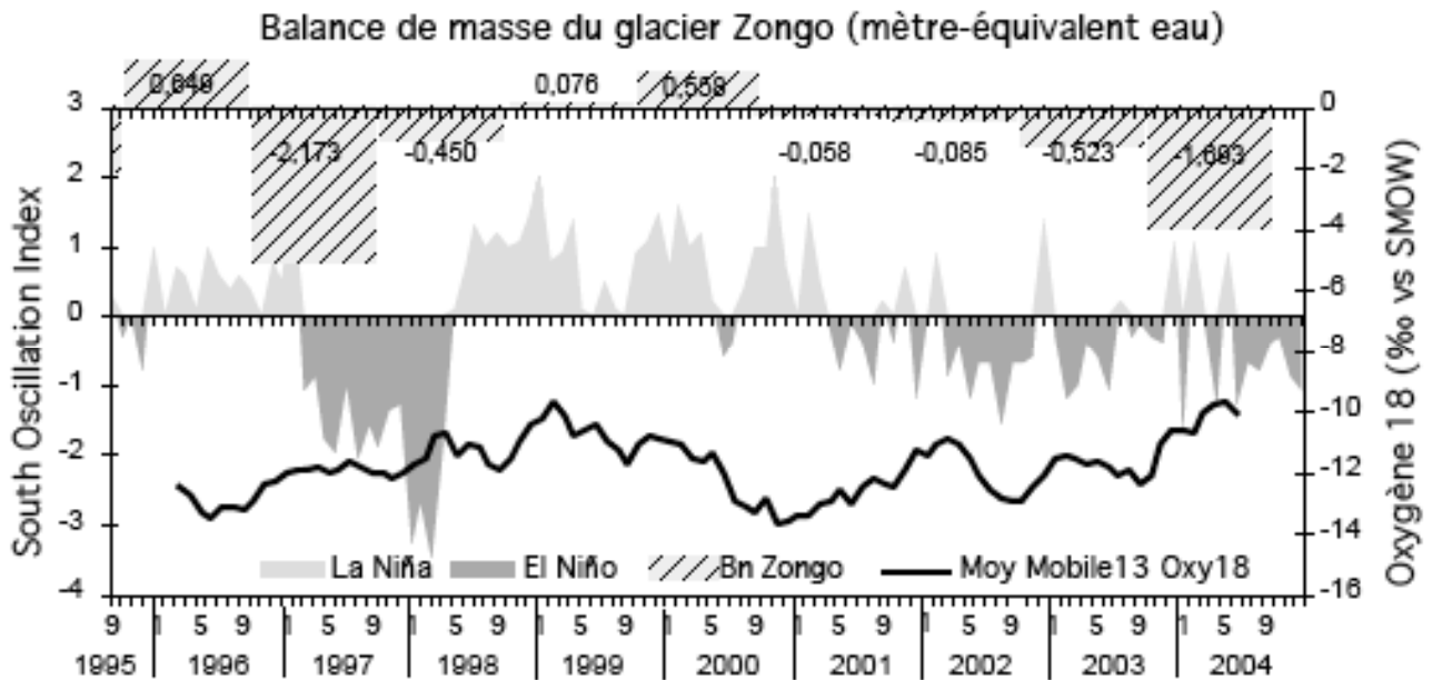
Fig. 8 Relation temporelle S.O.I. mensuels, balance nette annuelle du glacier Zongo et oxygène 18 (moyennes mobiles sur 13 mois pour ce dernier).
