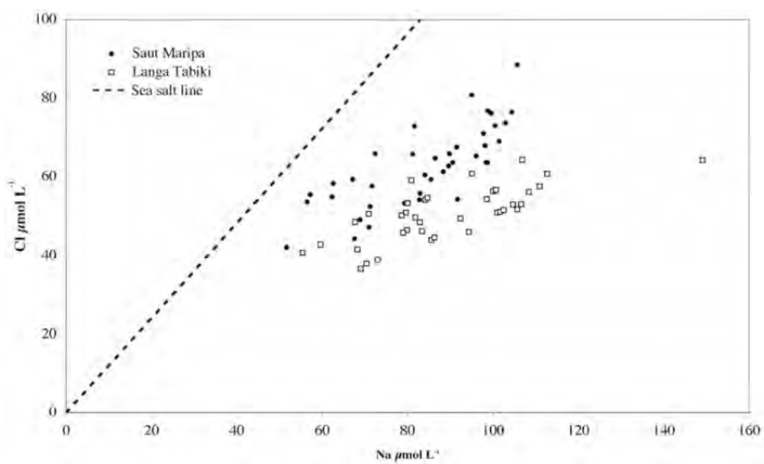
Fig. 9. Na / Cl ratio
