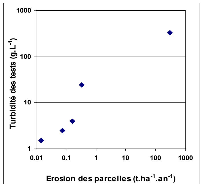
Figure 6: Relation entre turbidité des tests d'infiltrométrie et érosion mesurée sur parcelles d'érosion (2 années). Relation between turbidity of the infiltrometer tests and erosion measured on erosion plots (2 years).
